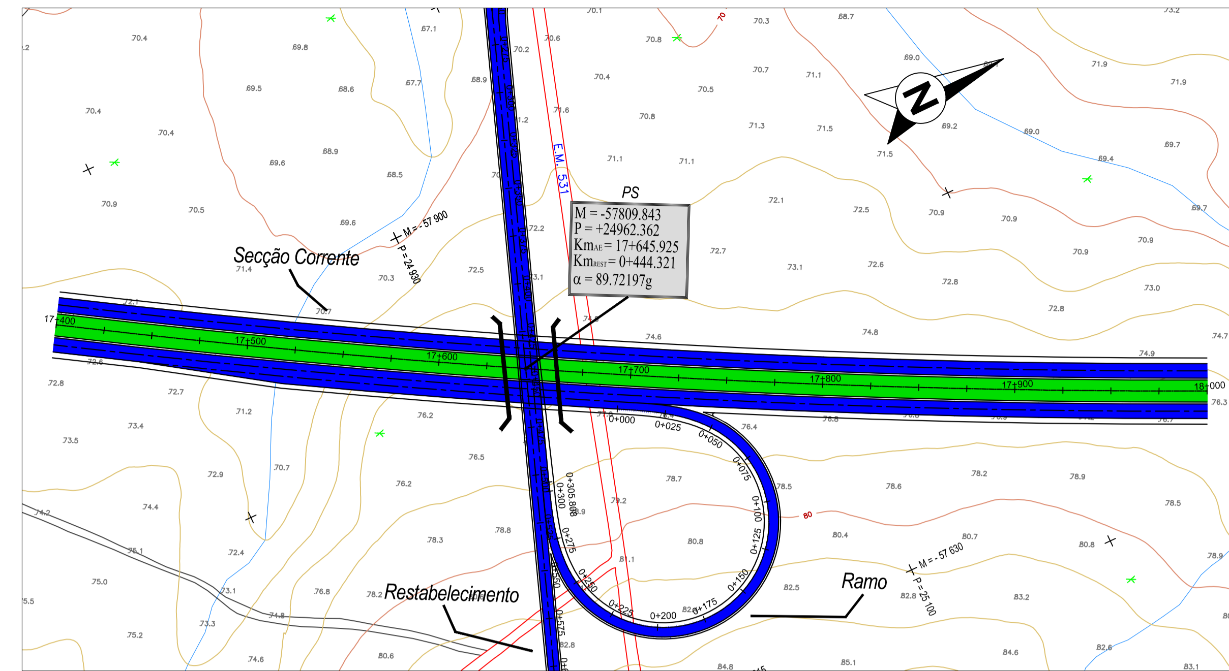
Planta Geral - Solução R=500
