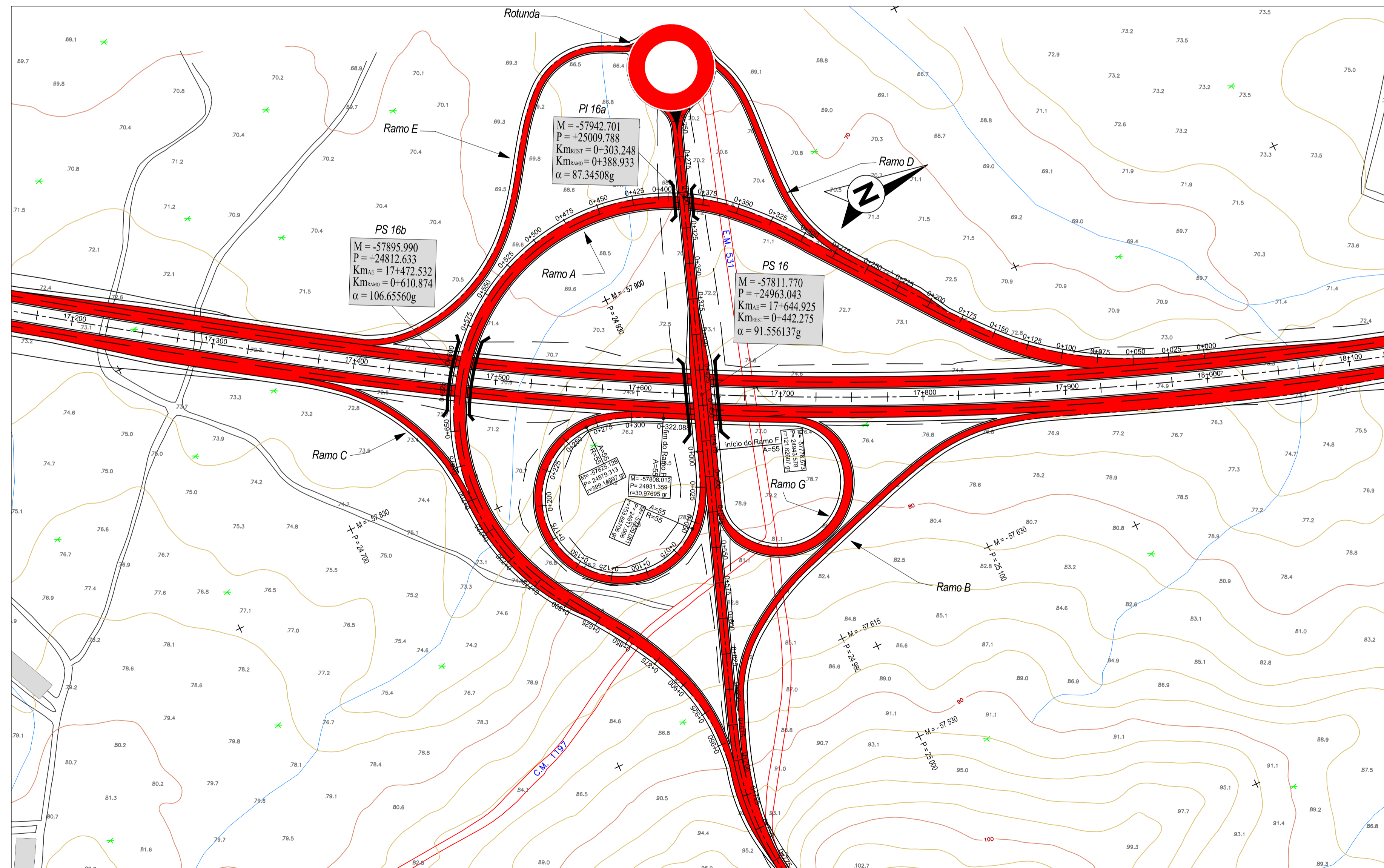
Planta Geral - Nó Inicial
