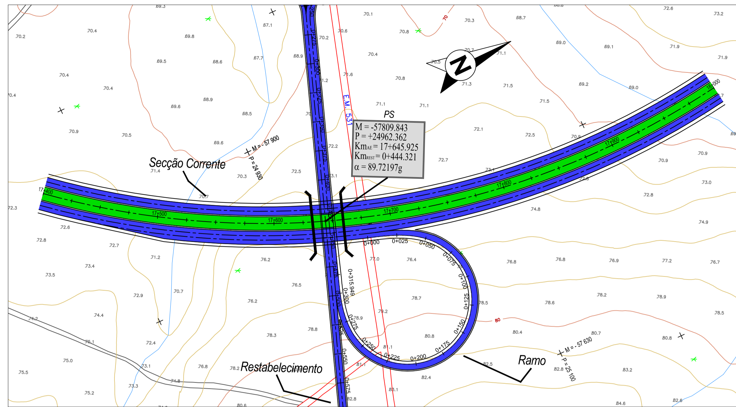
Planta Geral - Solução R=700
