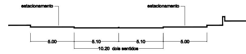
Perfil transversal da Rua Madre Teresa de Calcutá
