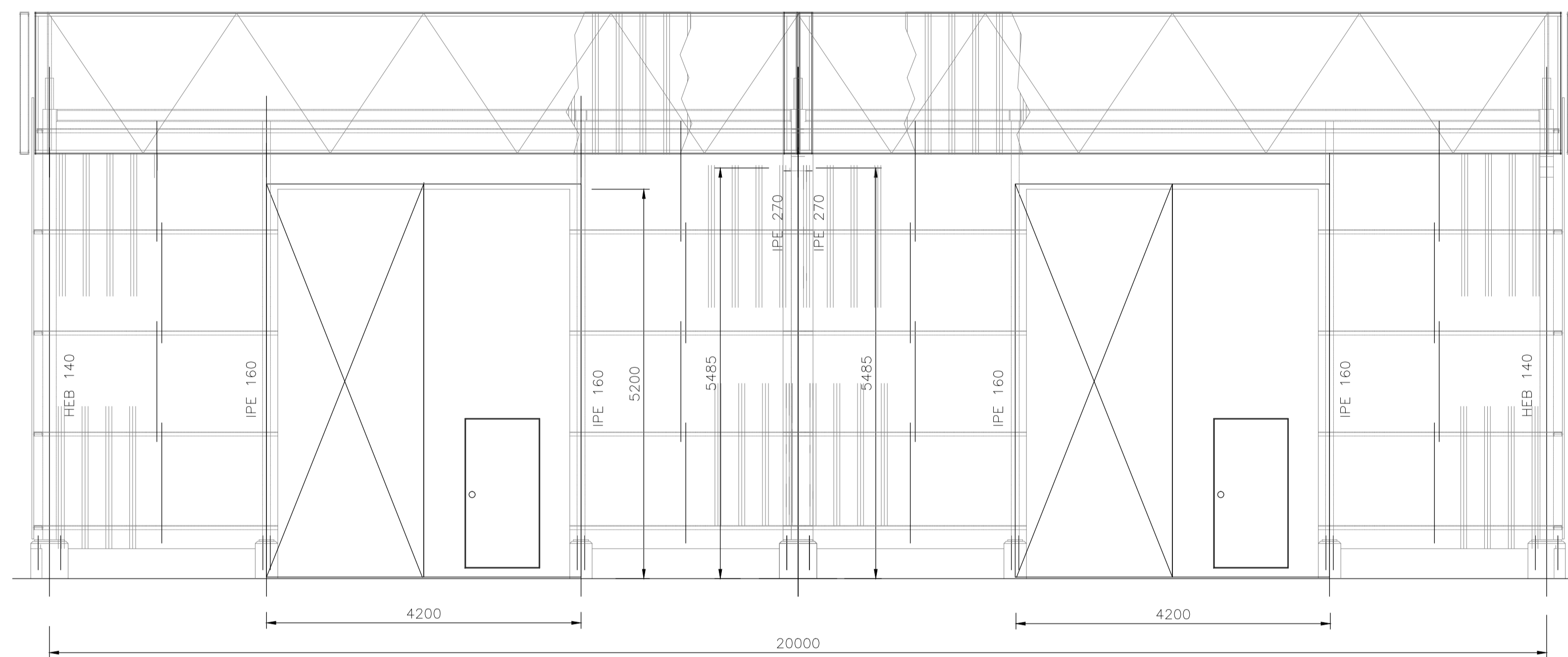
PÓRTICO-ALINHAMENTO A
