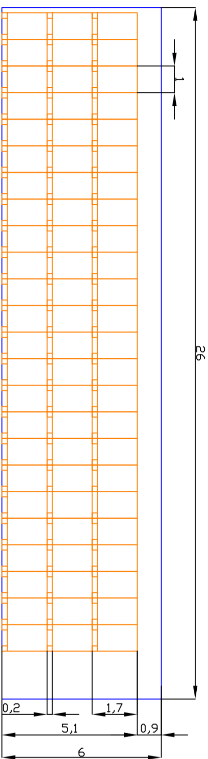
CORTE A-A
