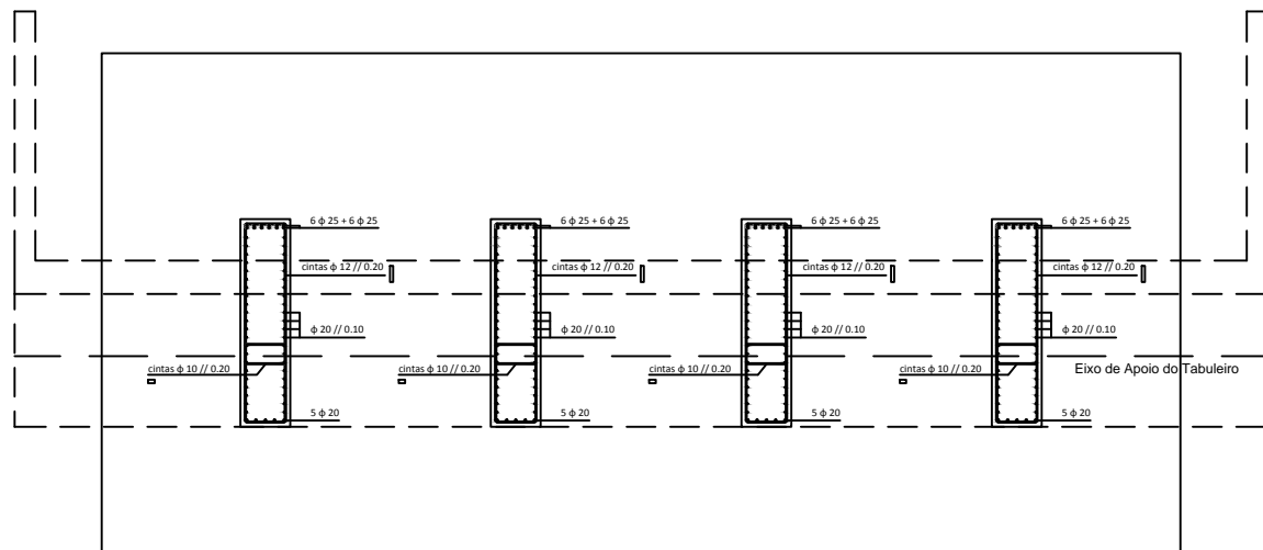
CORTE F-F A1 - 1/50 ; A3 - 1/100
