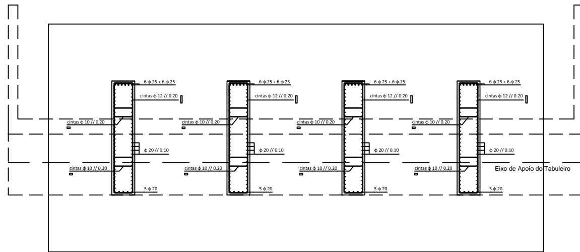
CORTE E-E A1 - 1/50 ; A3 - 1/100
