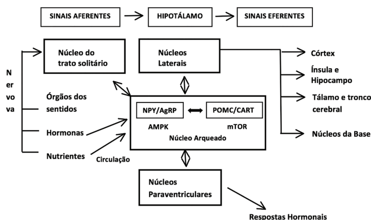
Figura 1. Representação esquemática da sinalização alimentar. NPY – Neuropéptido Y; AgRP – Proteína relacionada a agouti; POMC – Pró-opiomelanocortina; CART – Transcritos regulados por cocaína e anfetamina; AMPK – Proteína cinase dependente de AMP; mTOR – Proteína alvo da rapamicina em mamíferos (modificado de Damiani 11 ).
