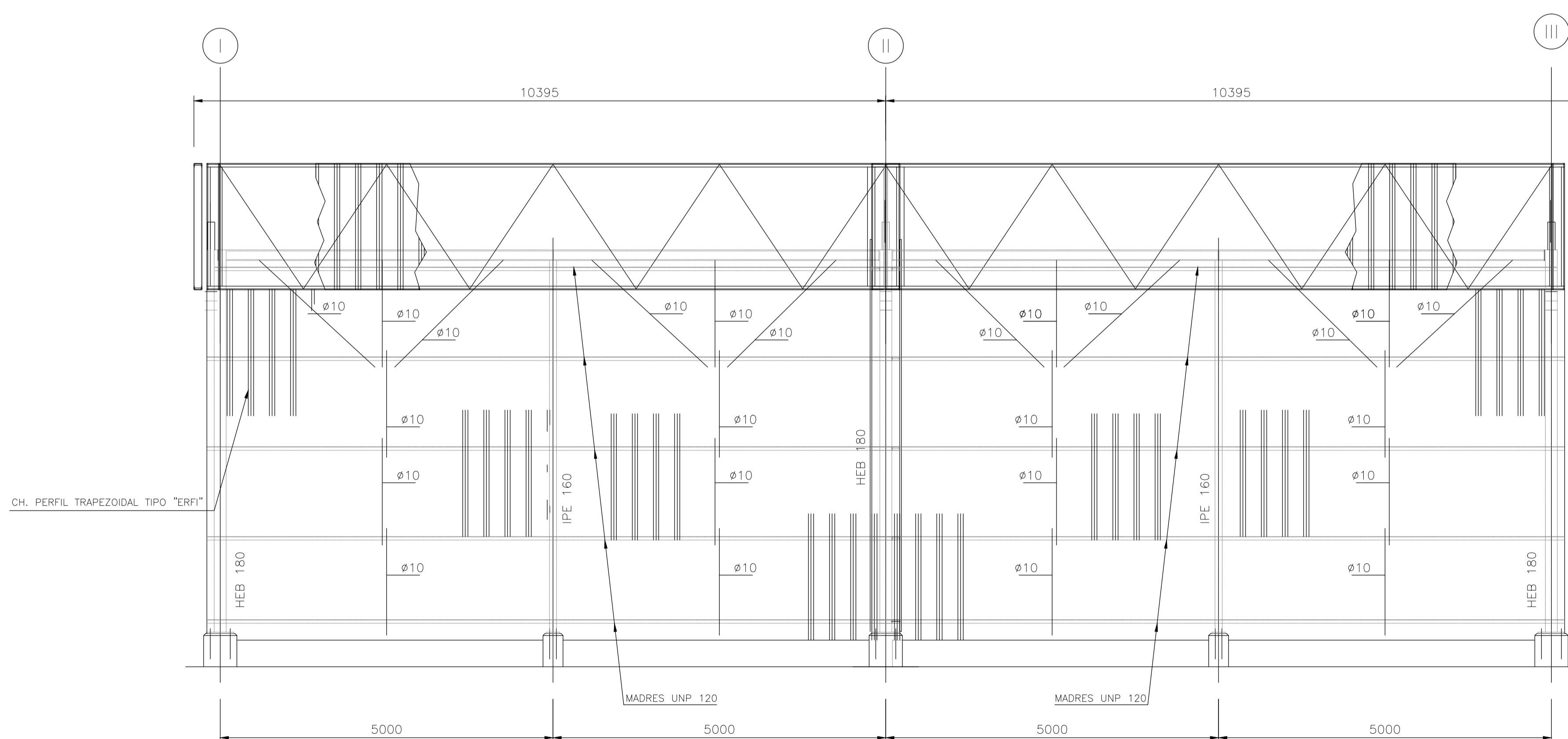
PÓRTICO-ALINHAMENTO C
