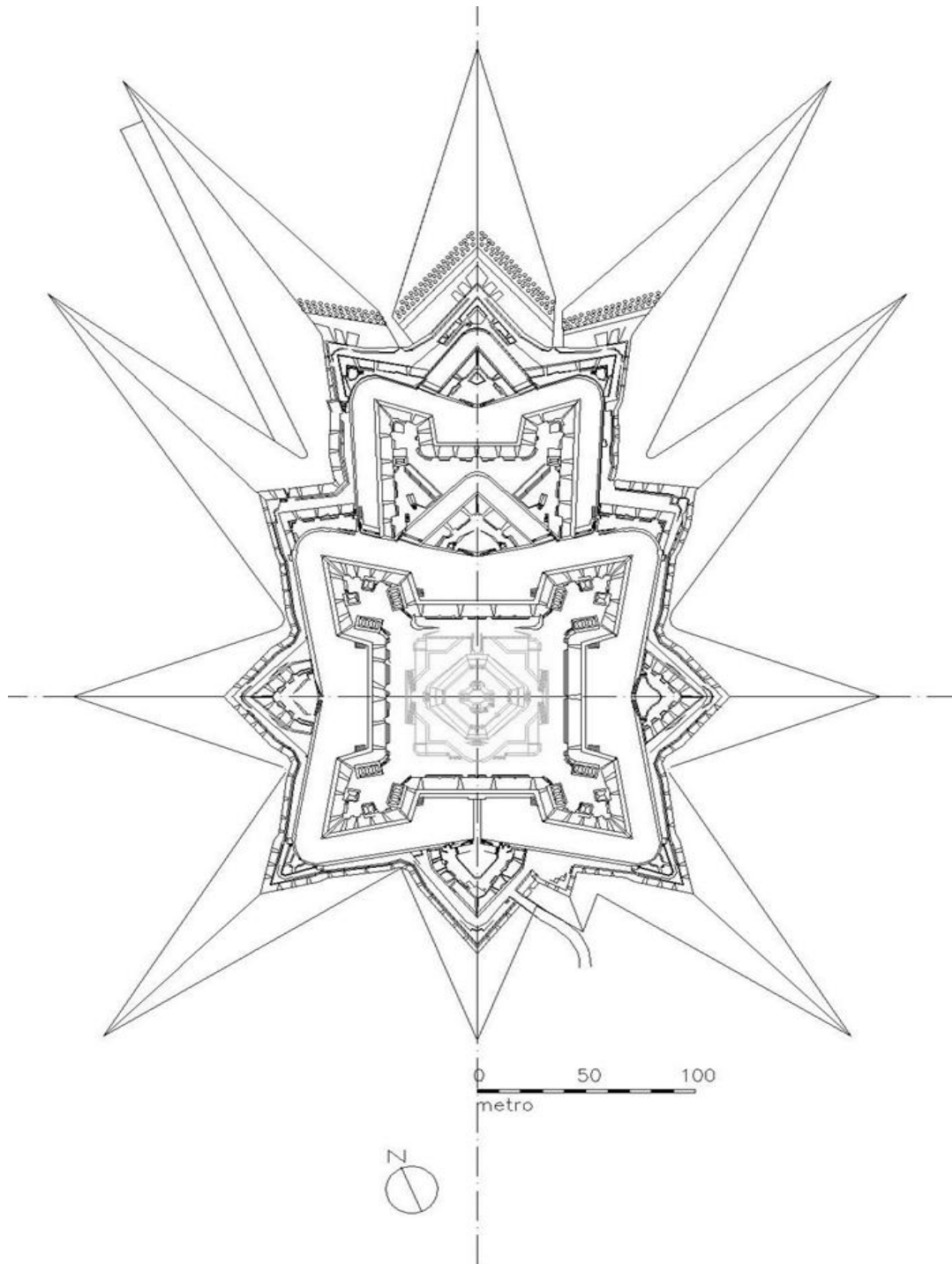
Planta Geral
