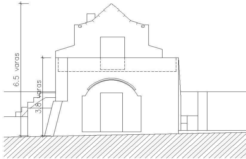
Quartéis - Alçado Principal
