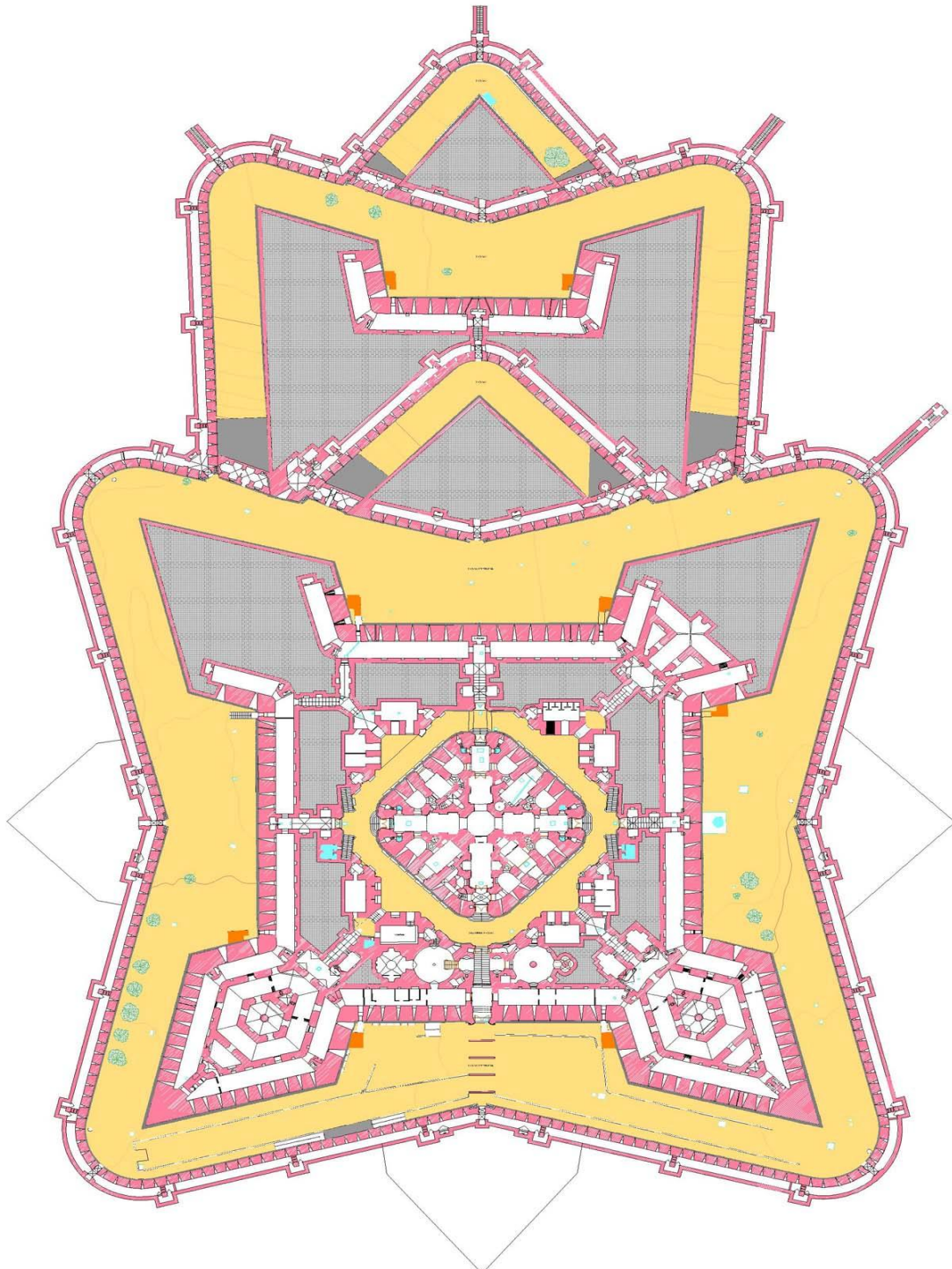
Planta Geral - piso 1 ( s/ escala)
