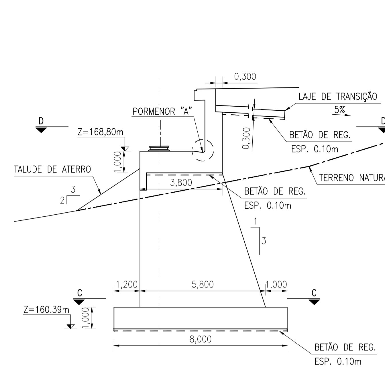
CORTE LONGITUDINAL ENCONTRO E2 (A1-1:100, A3-1:200)
