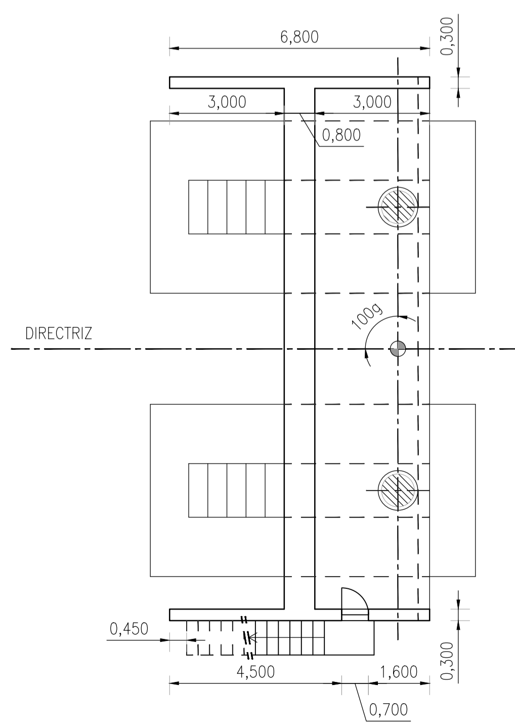
CORTE B-B (A1-1:100, A3-1:200)
