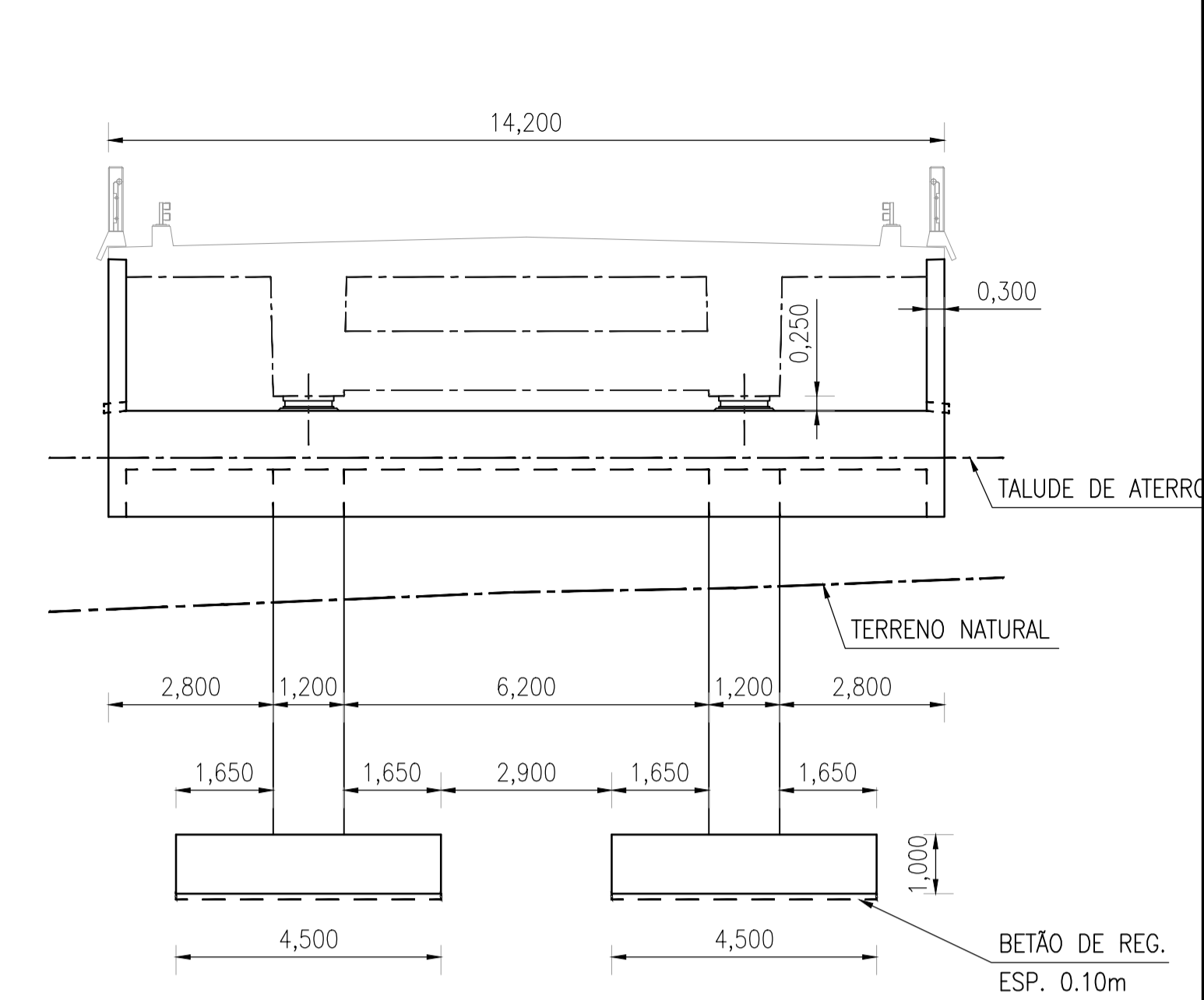
ALÇADO ENCONTRO SUL (A1-1:100, A3-1:200)
