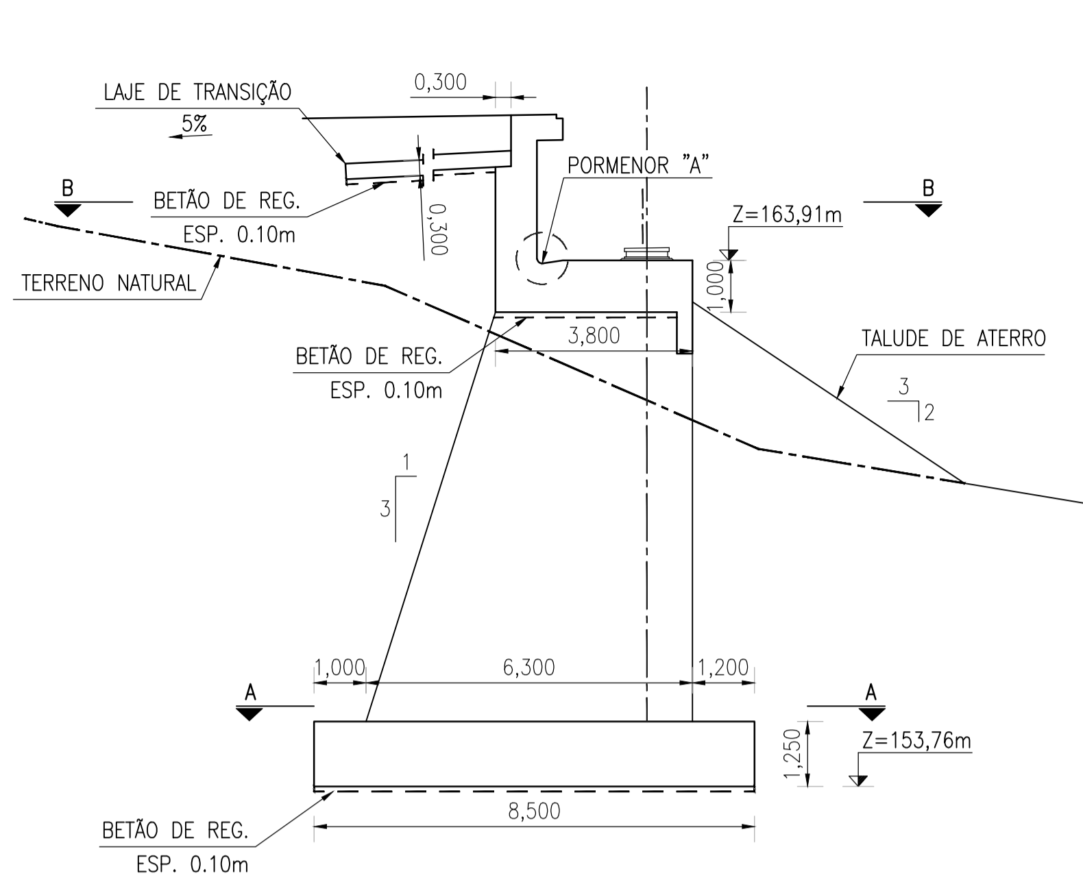
CORTE LONGITUDINAL ENCONTRO E1 (A1-1:100, A3-1:200)
