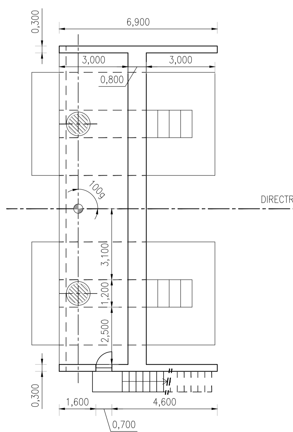
CORTE D-D (A1-1:100, A3-1:200)
