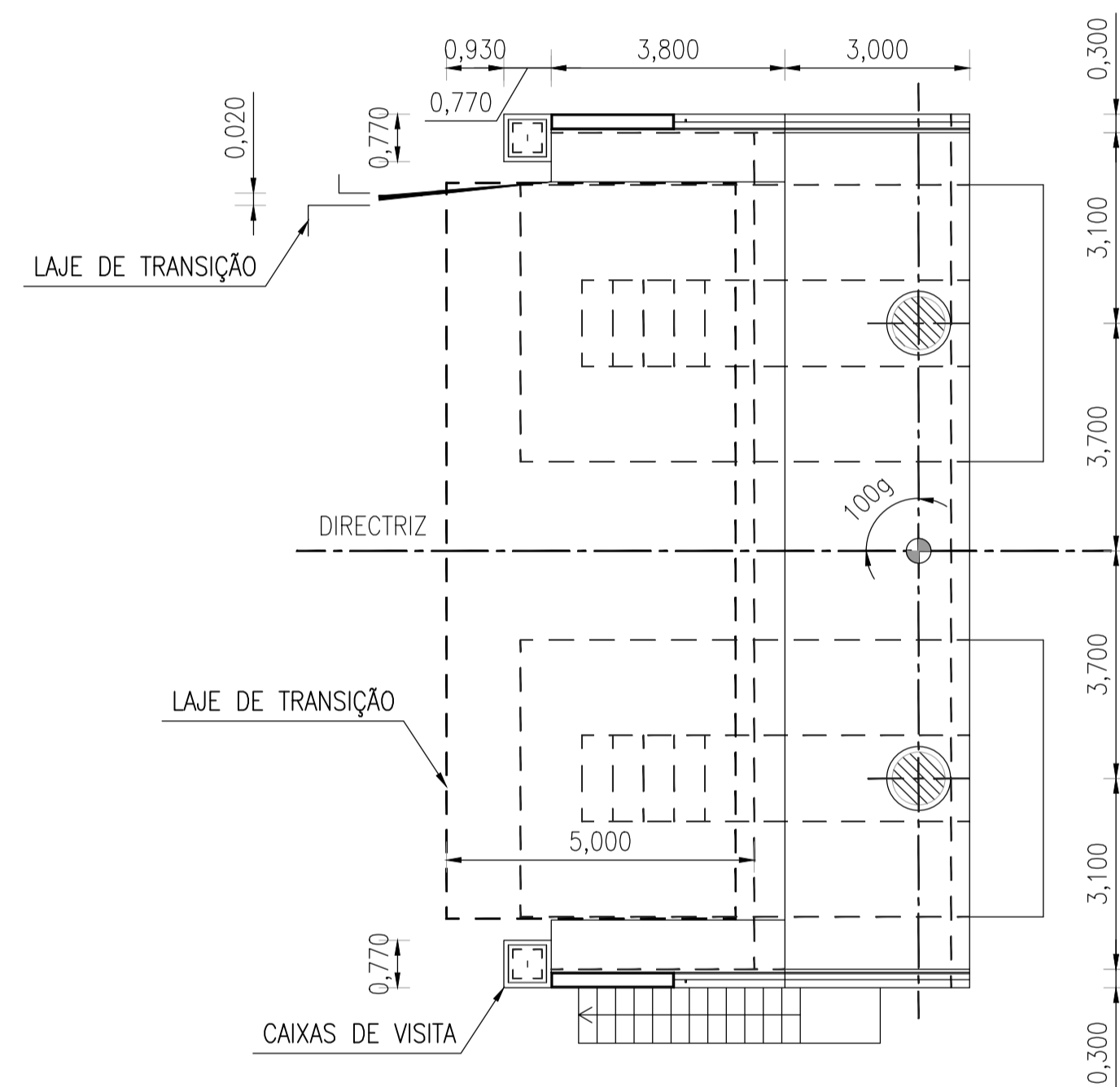
PLANTA ENCONTRO E1 (A1-1:100, A3-1:200)
