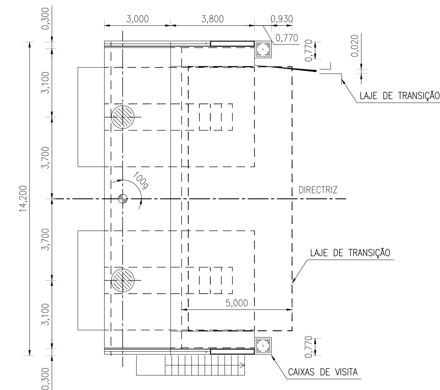
PLANTA ENCONTRO E2 (A1-1:100, A3-1:200)
