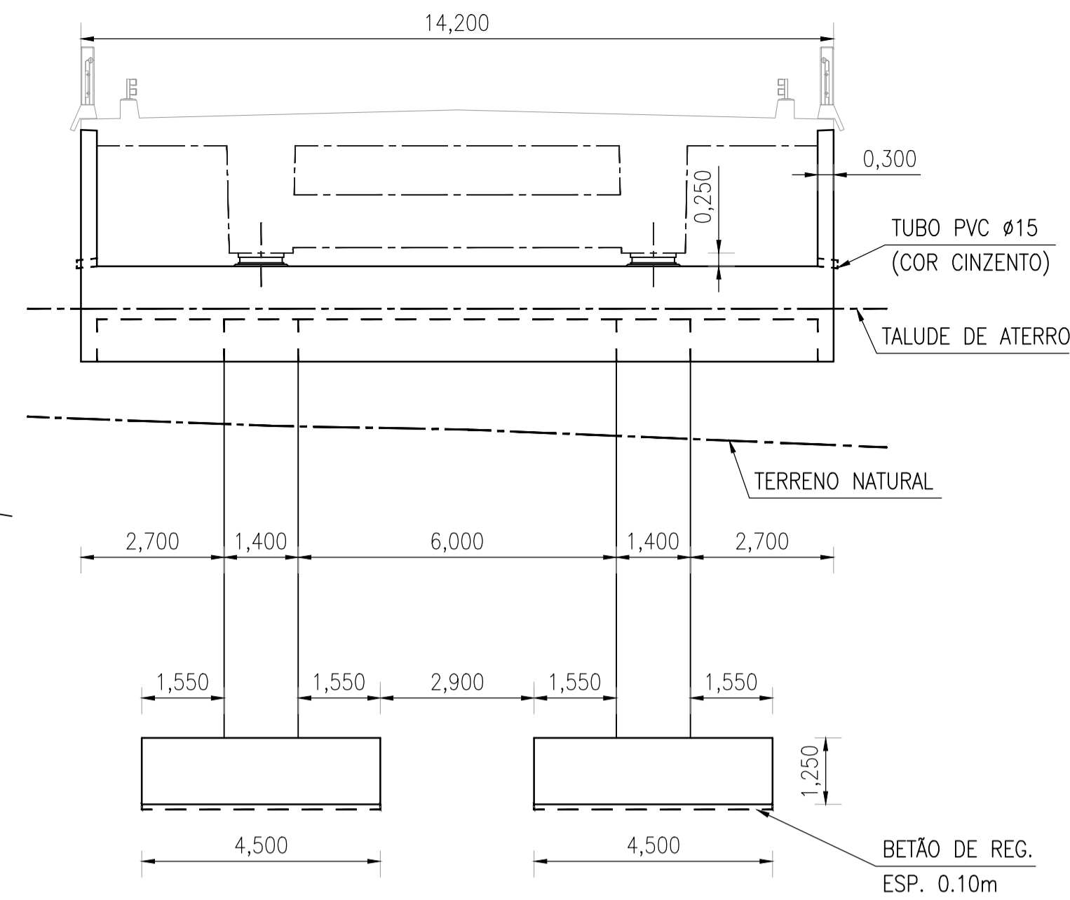
ALÇADO ENCONTRO NORTE (A1-1:100, A3-1:200)
