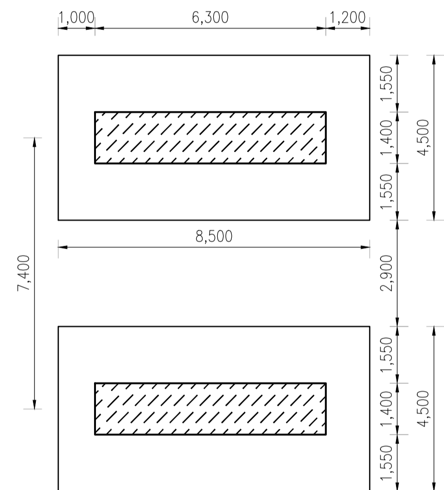
CORTE A-A (A1-1:100, A3-1:200)
