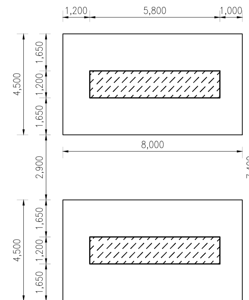
CORTE C-C (A1-1:100, A3-1:200)
