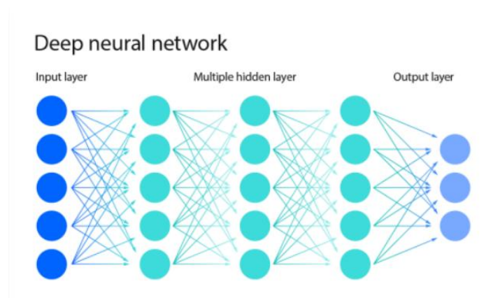
Figura 2.11: Redes Neurais
