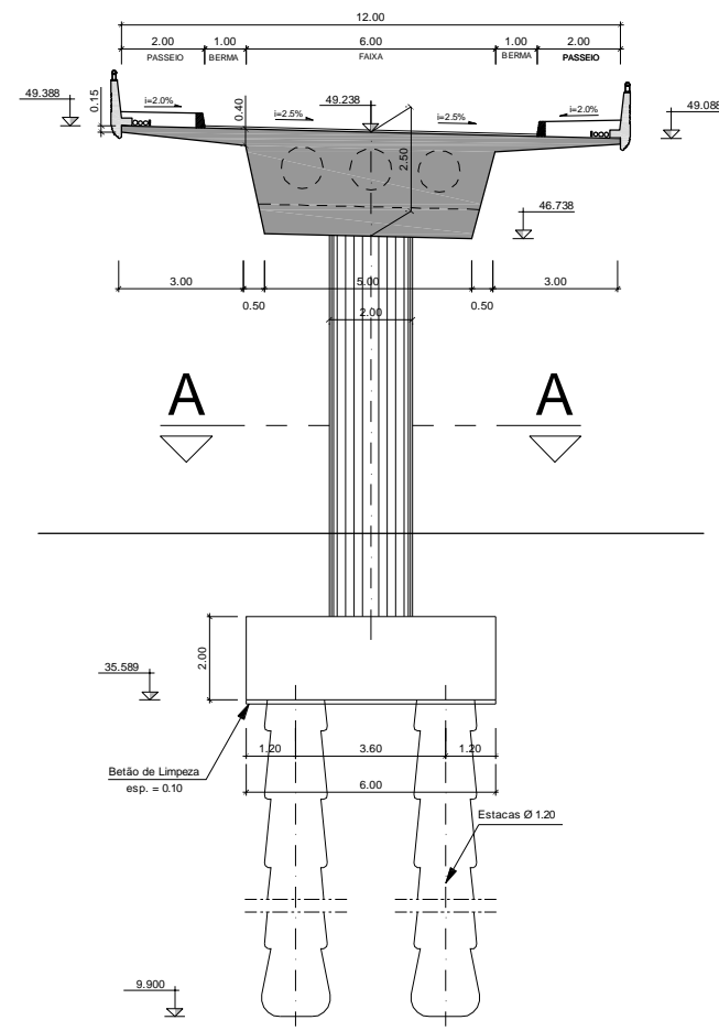
CORTE TRANSVERSAL - PILAR 3 ESC.=1:200
