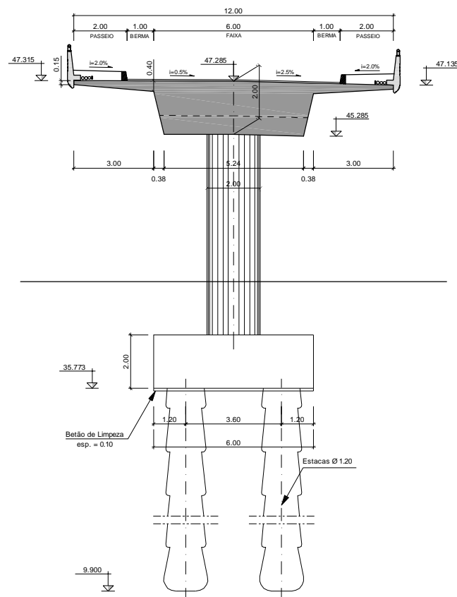
CORTE TRANSVERSAL - PILAR 2 ESC.=1:200
