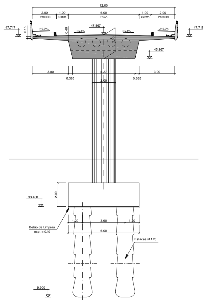
CORTE TRANSVERSAL - PILAR 5 ESC.=1:200
