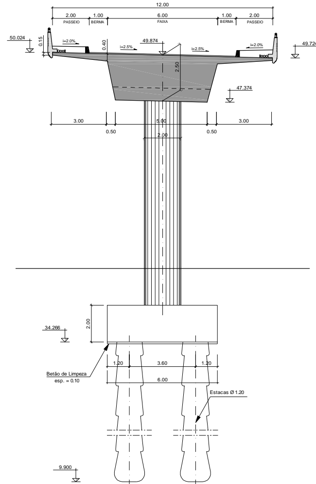
CORTE TRANSVERSAL - PILAR 4 ESC.=1:200
