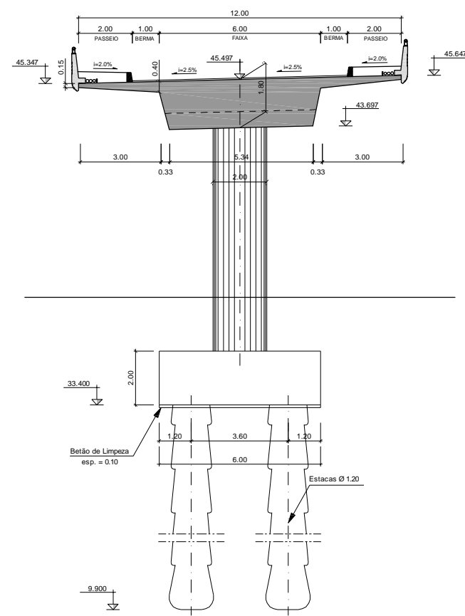
CORTE TRANSVERSAL - PILAR 6 ESC.=1:200
