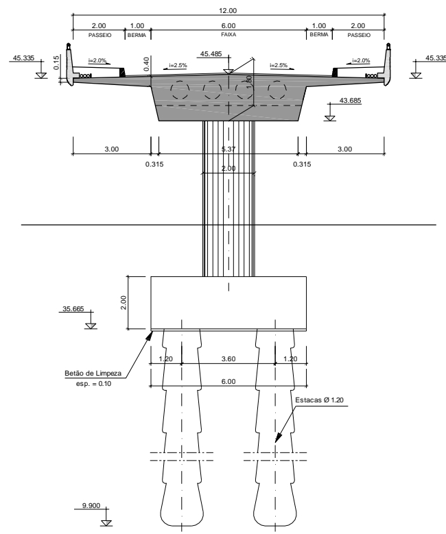
CORTE TRANSVERSAL - PILAR 1 ESC.=1:200
