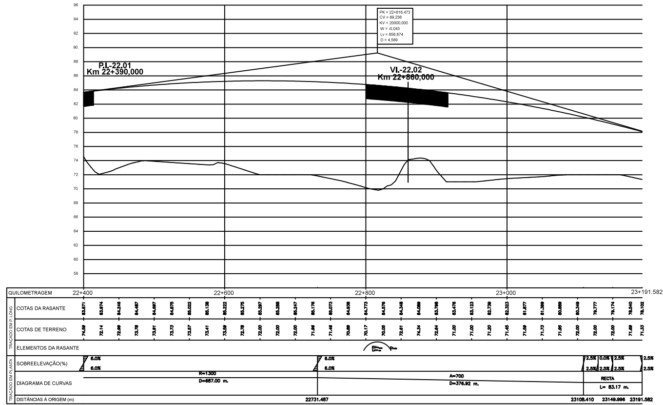
PERFIL LONGITUDINAL: VIA PRINCIPAL
