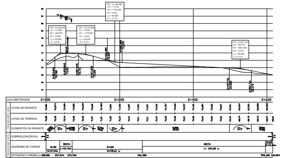
PERFIL LONGITUDINAL: RESTABELECIMENTO
