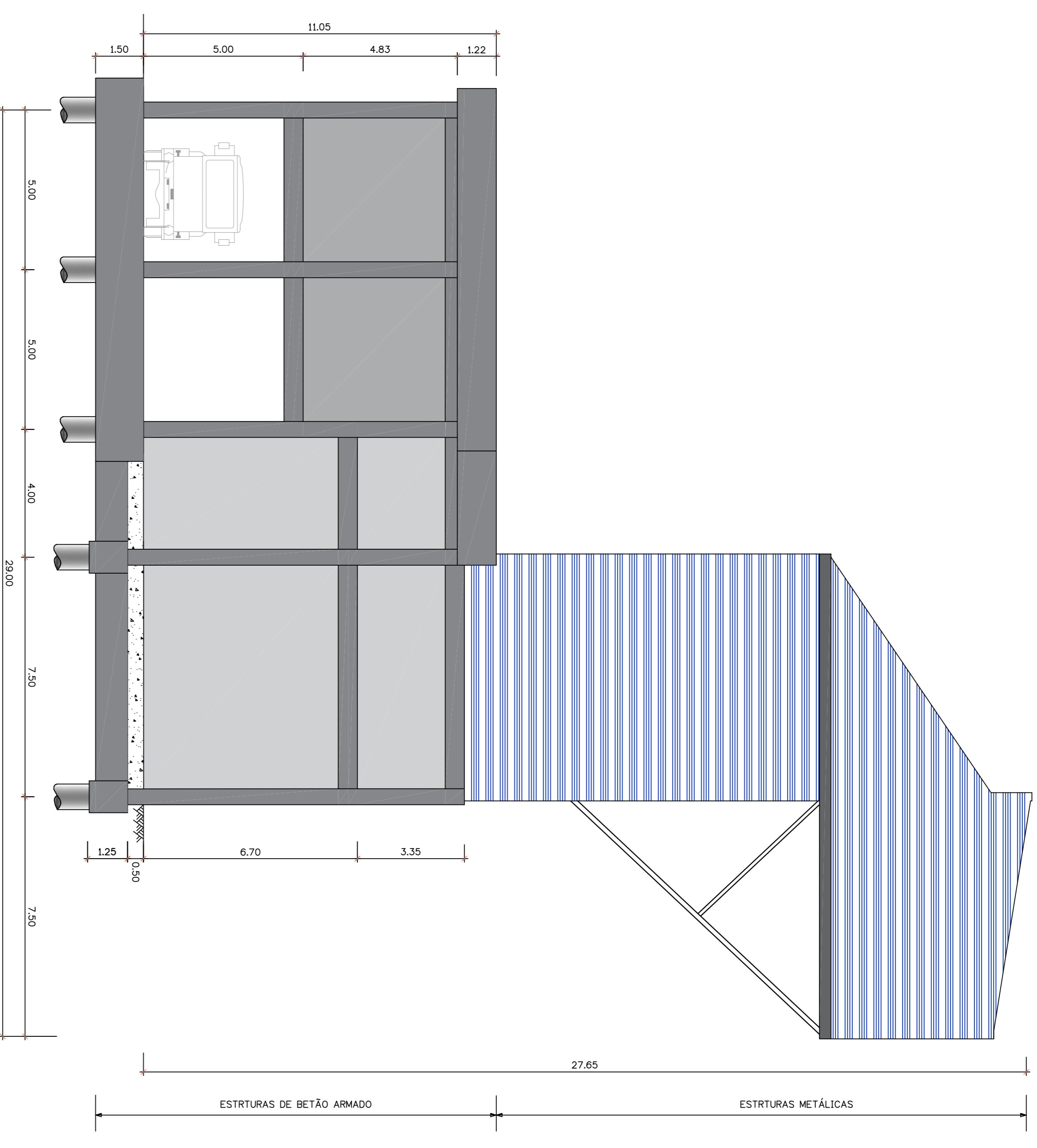
ALÇADO LATERAL DIREITO
