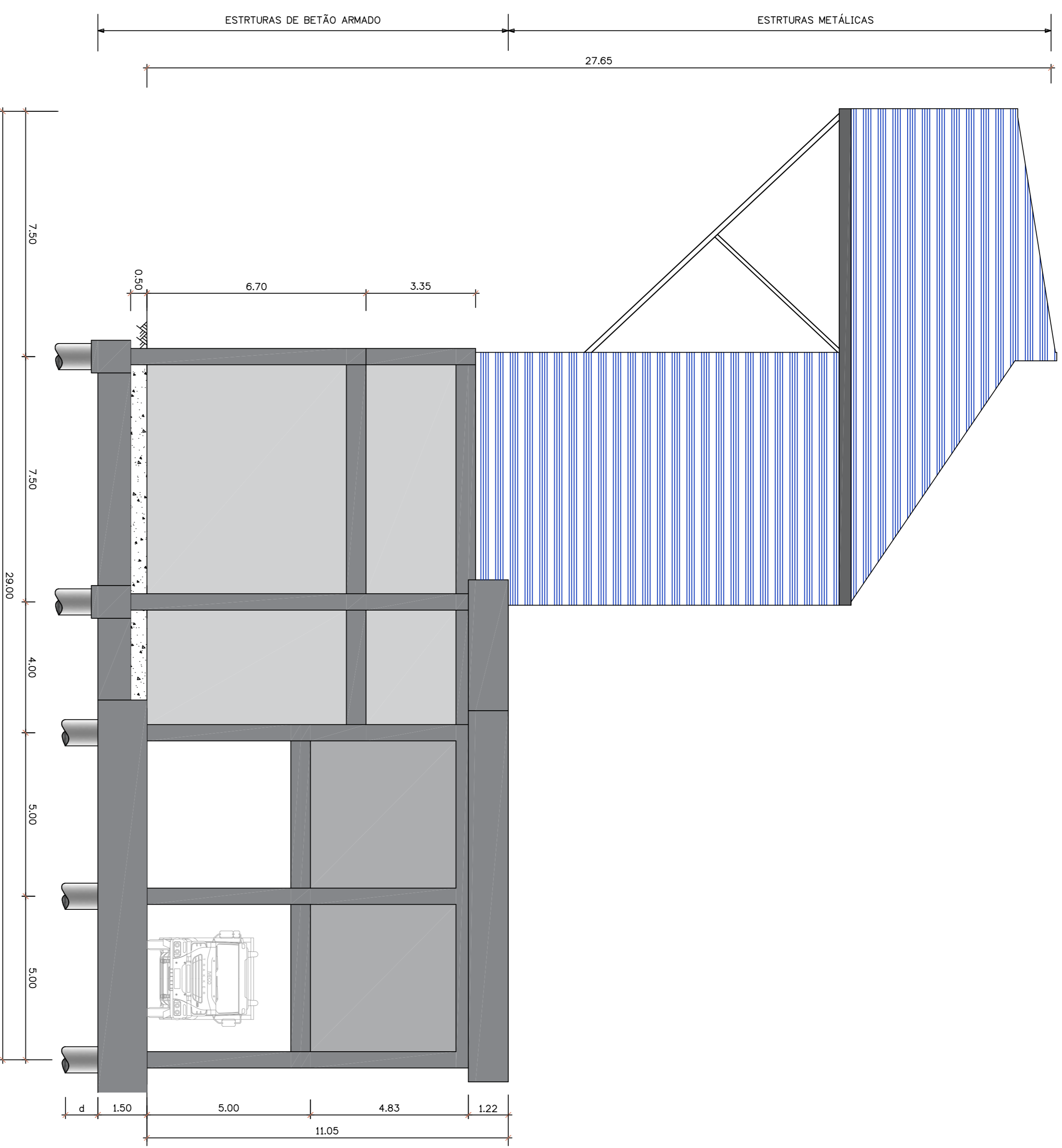
ALÇADO LATERAL ESQUERDO
