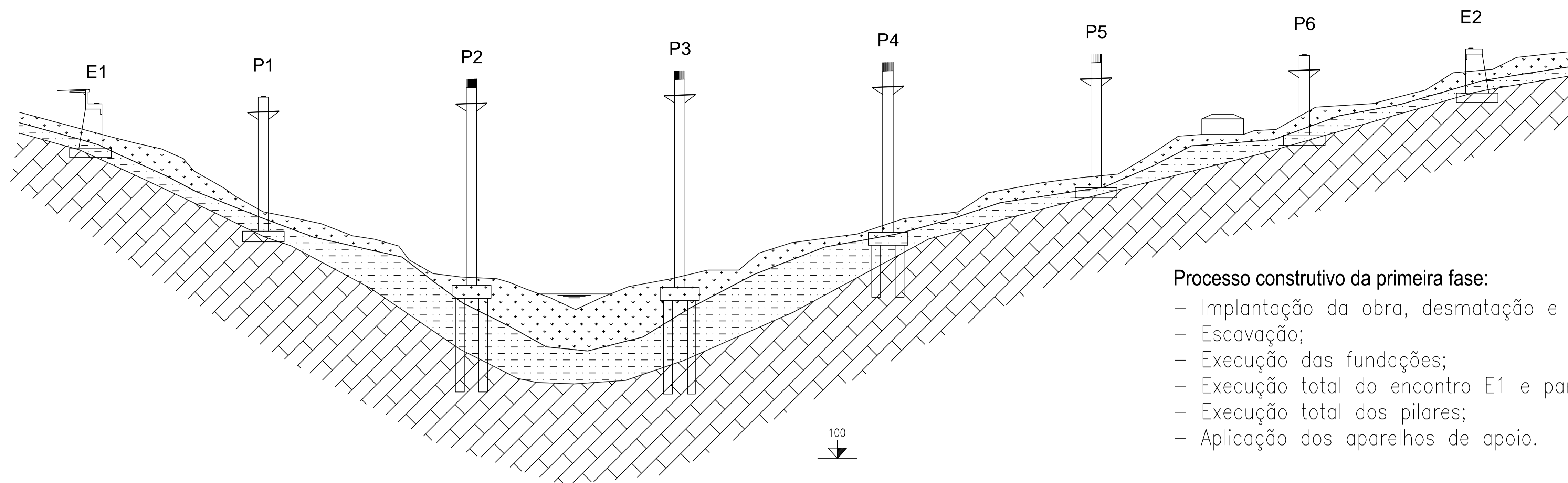
Primeira Fase ESCALA - 1:500
