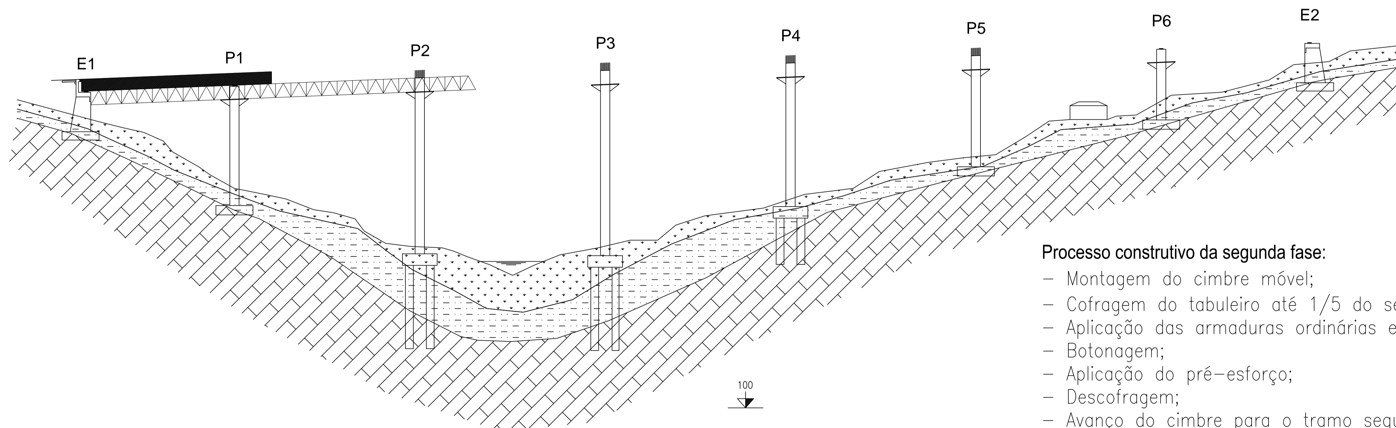
Segunda Fase ESCALA - 1:500
