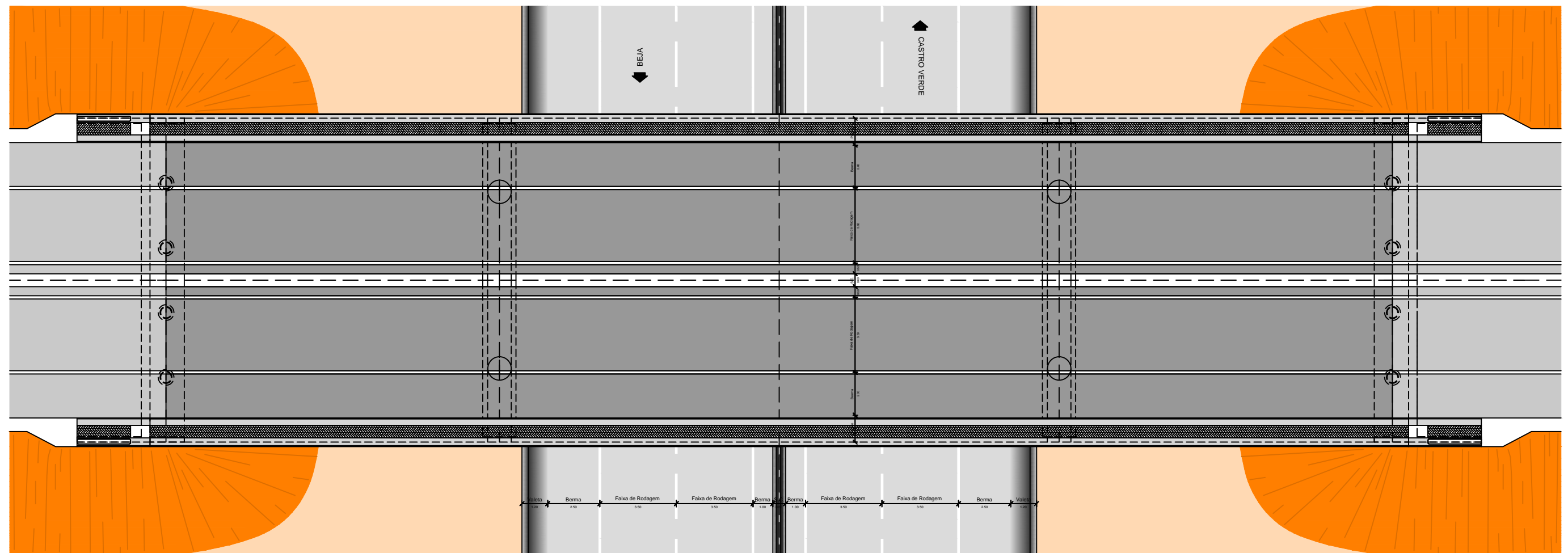
PLANTA A1 - 1/100 ; A3 - 1/200
