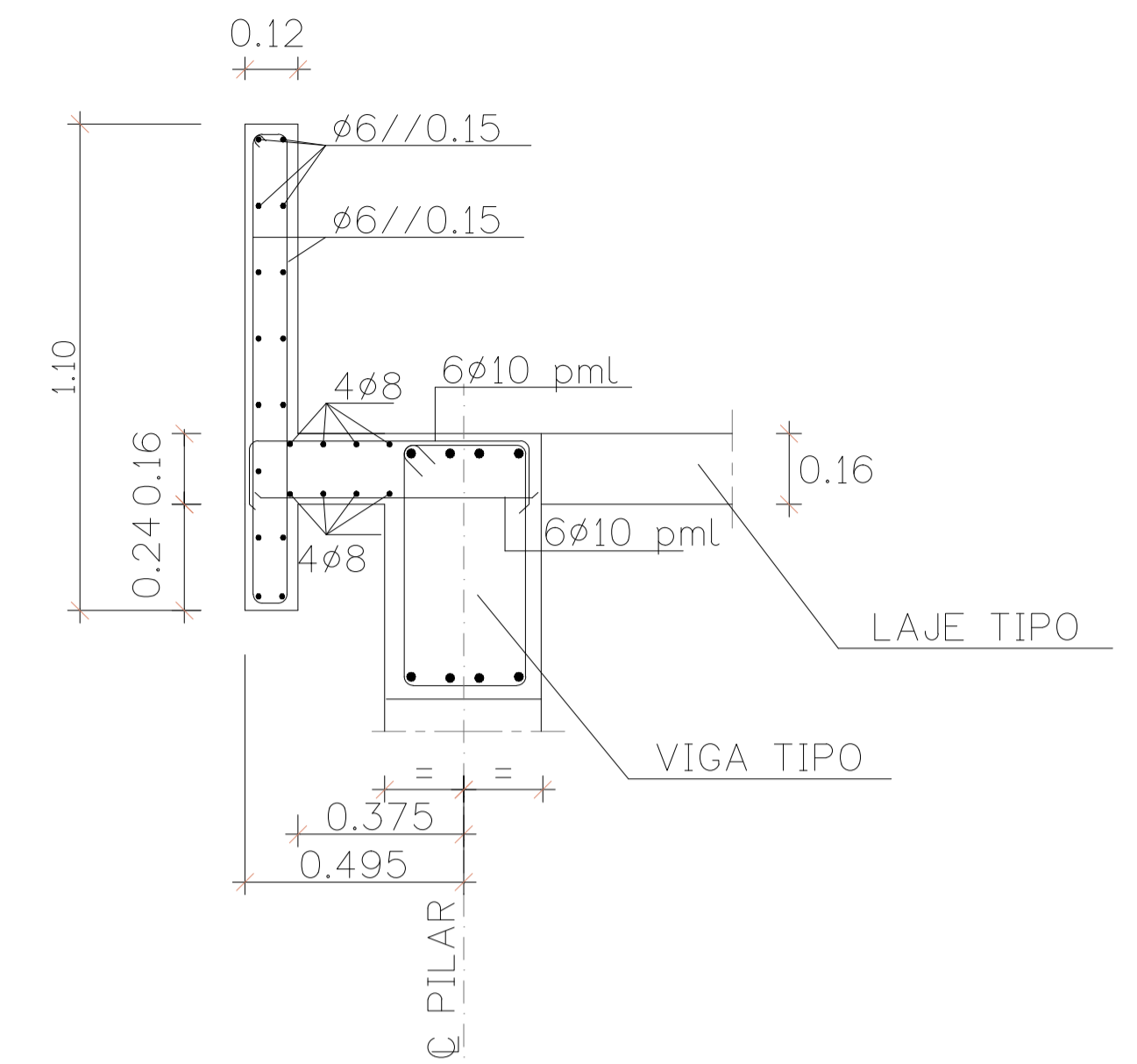
CORTE TIPO - ARMADURAS PLATIBANDAS
