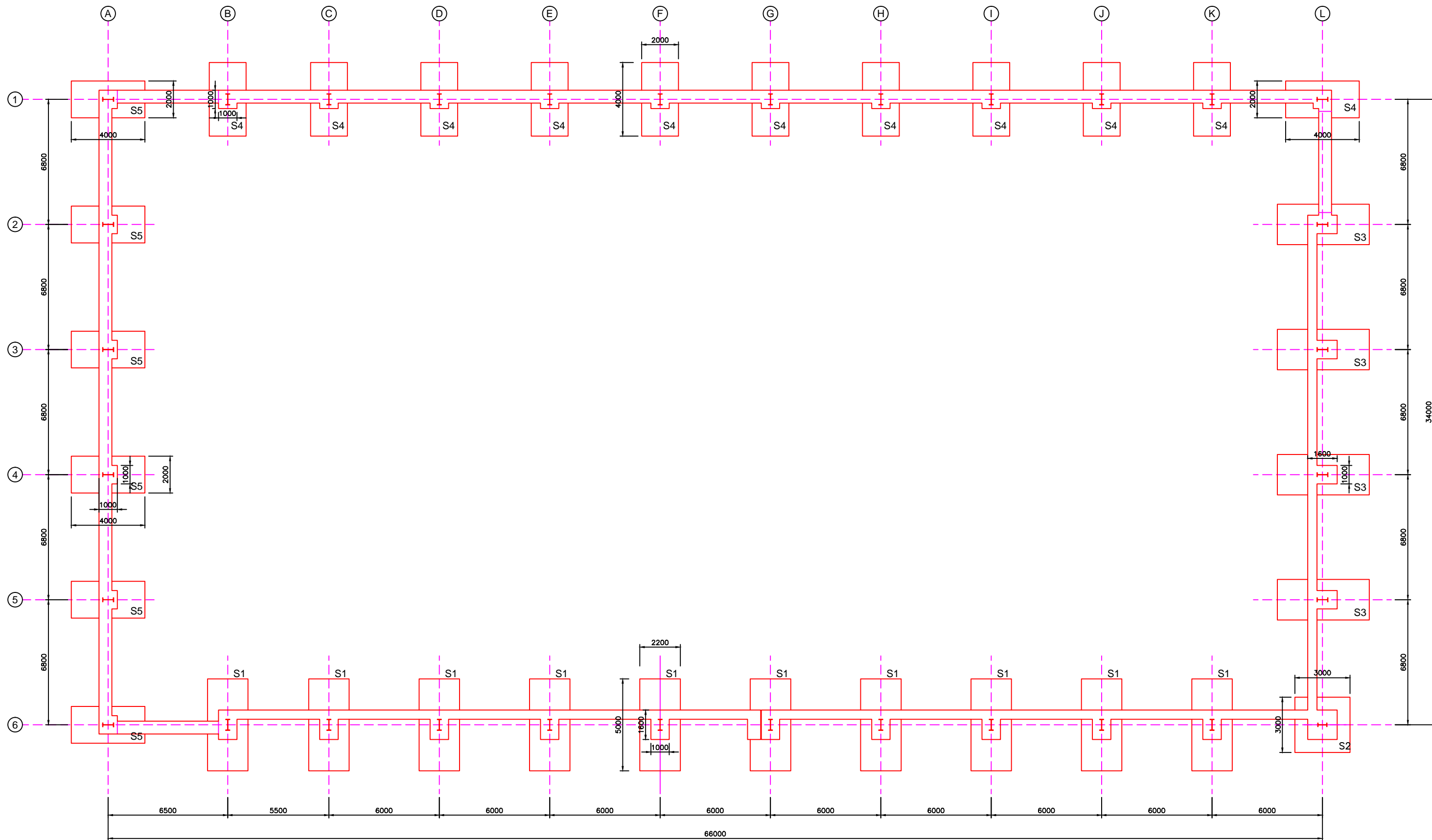
PLANTA DAS FUNDAÇÕES
