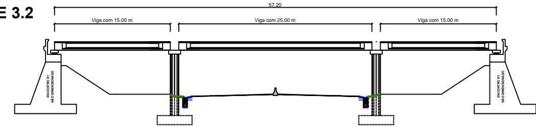
COLOCAÇÃO DAS VIGAS PRÉ-FABRICADAS NO VÃO CENTRAL
