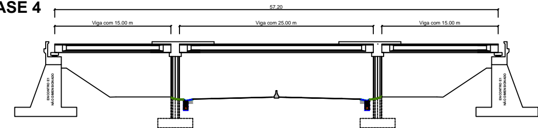
CONSTRUÇÃO DAS RESTANTES PARTES DAS CARLINGAS APLICAÇÃO DE BETÃO ATÉ AO 1/5 DE VÃO, COMO SE INDICA APLICAÇÃO DO PRÉ-ESFORÇO DE CONTINUIDADE
