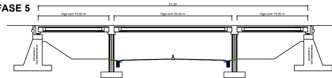
APLICAÇÃO DO BETÃO PARA CONSTRUÇÃO DA LAJE NA RESTANTE ÁREA DO TABULEIRO
