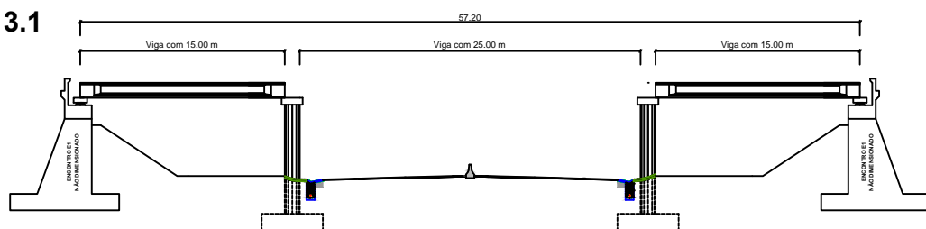
COLOCAÇÃO DAS VIGAS PRÉ-FABRICADAS NOS VÃOS EXTREMOS
