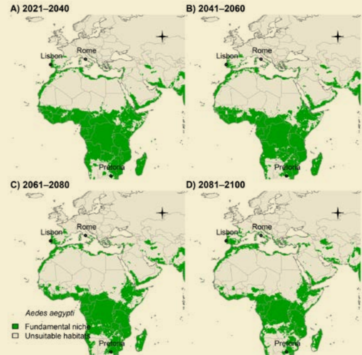
(A) 2021-2040; (B) 2041-2060; (C) 2061-2080; e (D) 2081-2100. Projeções climáticas futuras baseadas no modelo climático global GFDL-ESM4.1 da NOAA no caminho socioeconómico partilhado SSP3-7.0 de rivalidade regional. As localizações das capitais dos países foram mostradas para referência.
