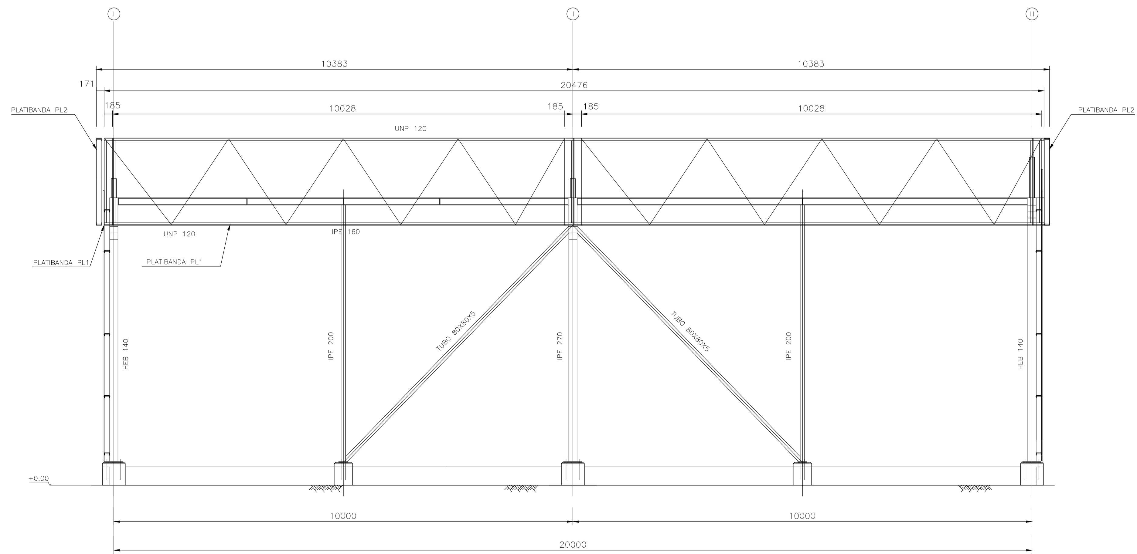
PÓRTICO - ALINHAMENTO C
