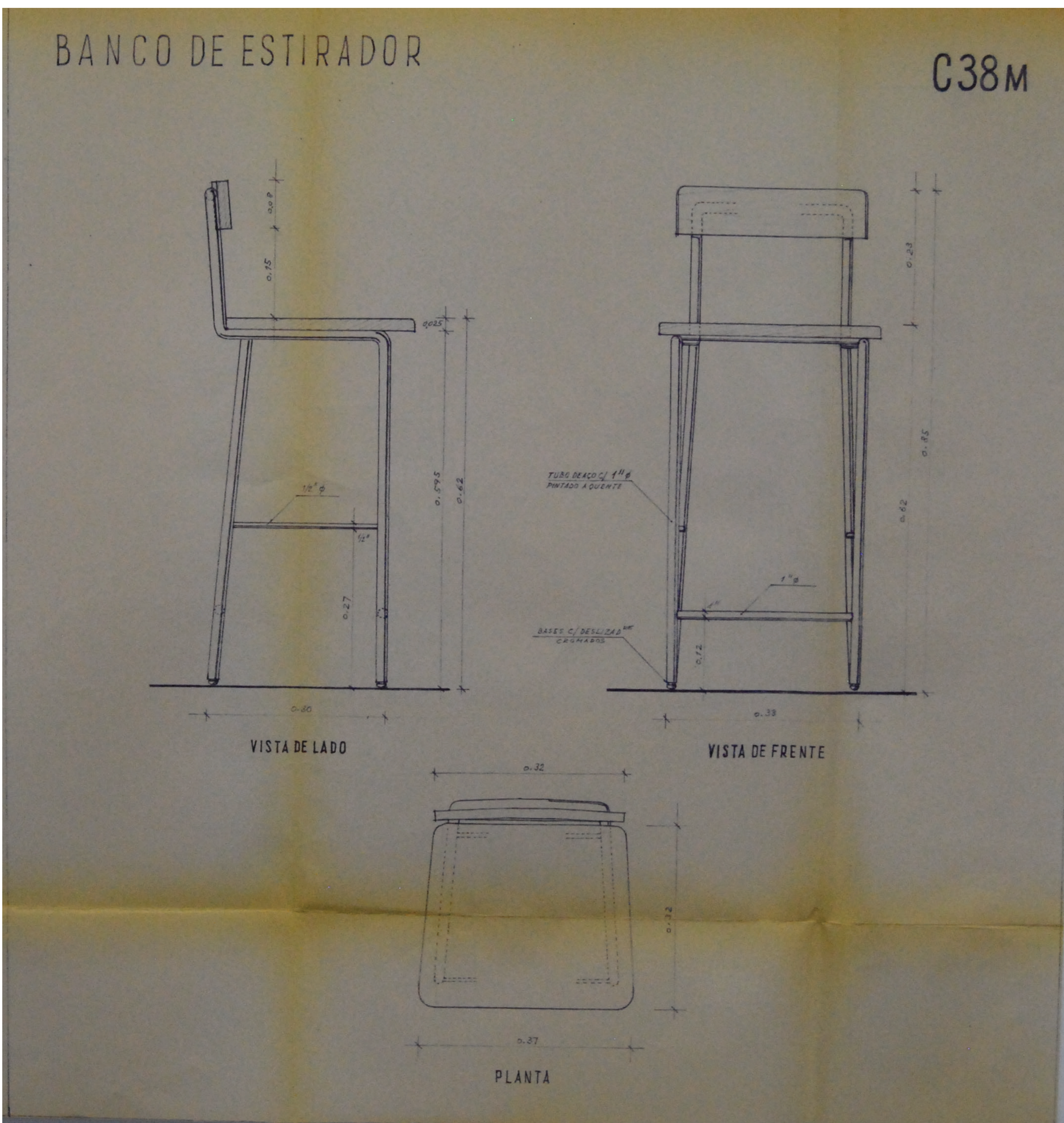
Banco de estirador © Arquivo do ISEL
