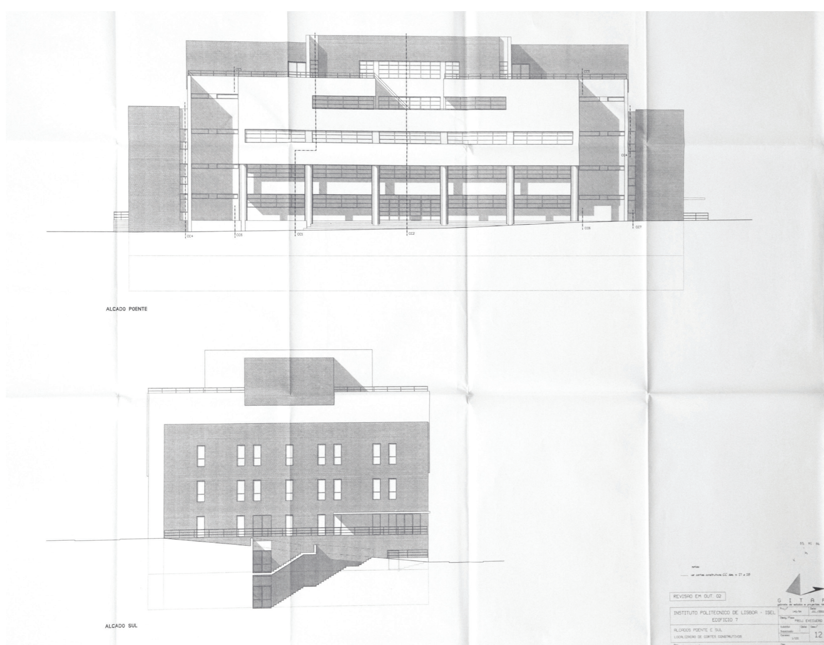
Projeto Alçado Poente de 2002 © Arquivo ISEL
