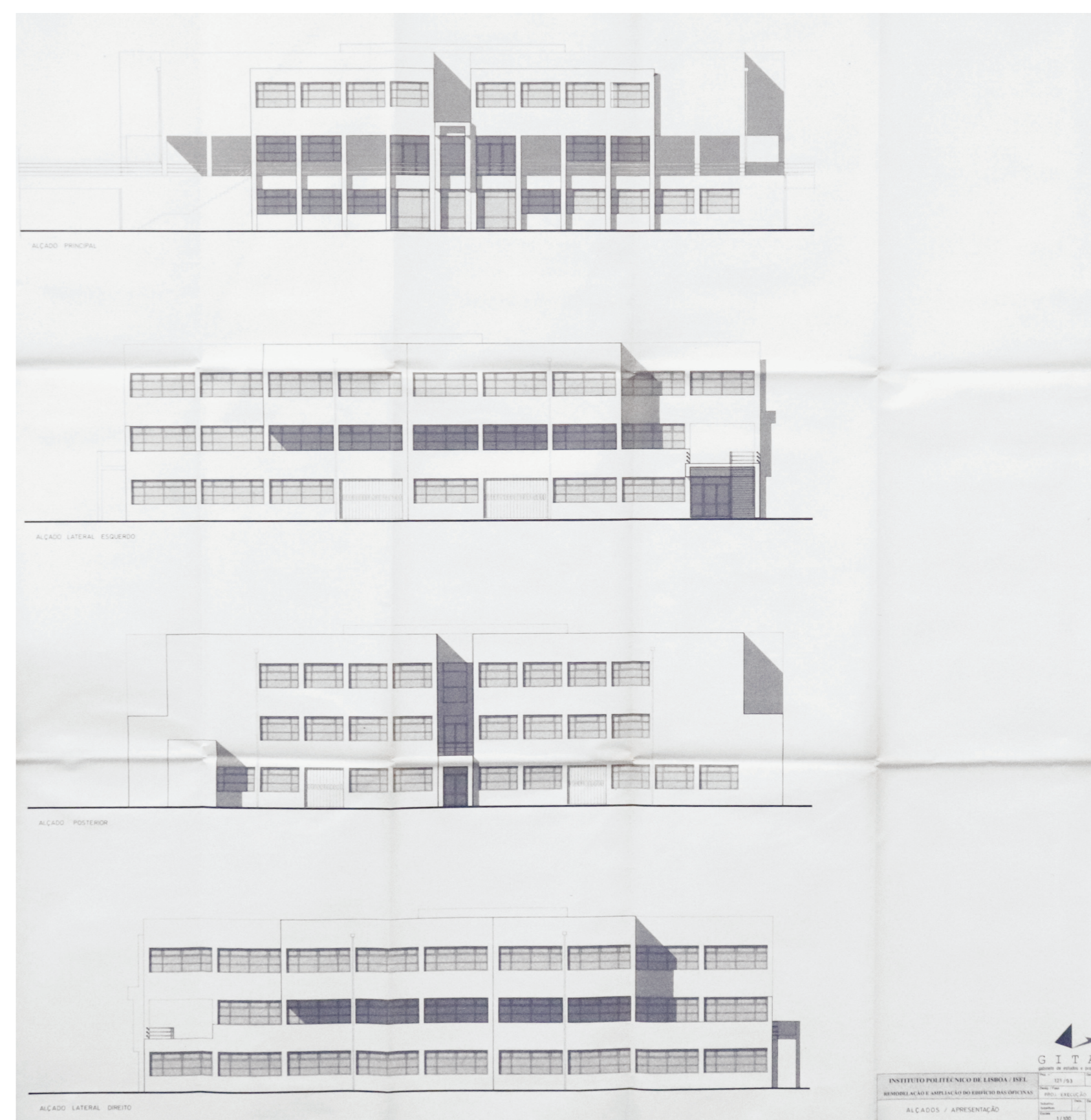
Projeto Alçado Principal, 1993 © Arquivo ISEL
