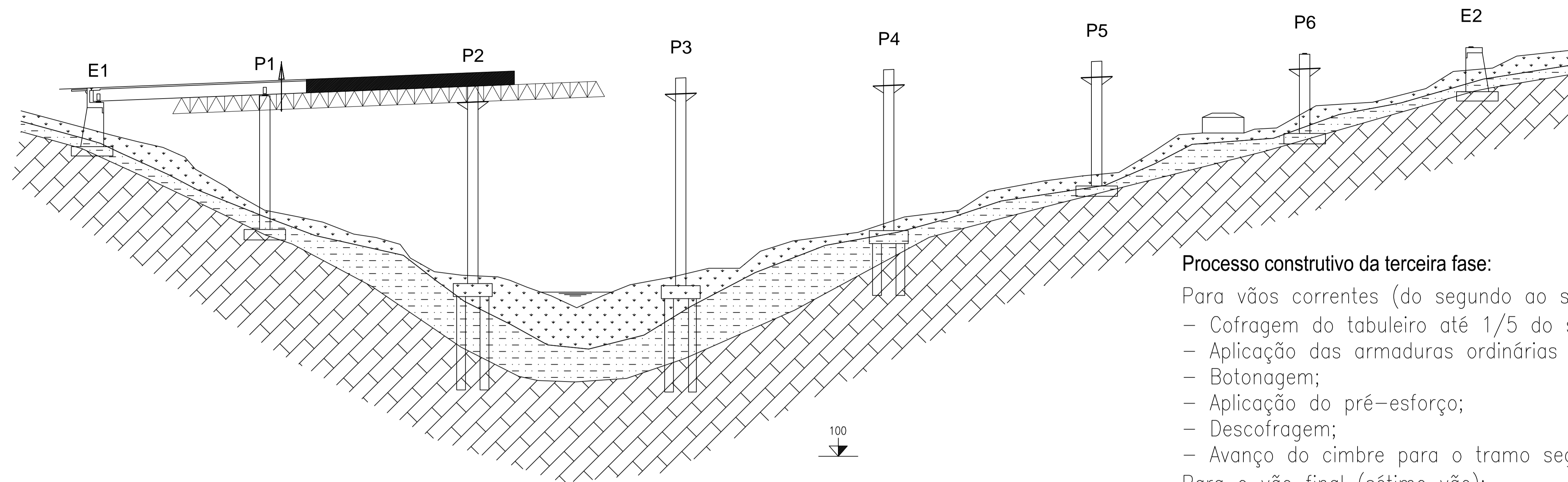
Terceira Fase ESCALA - 1:500
