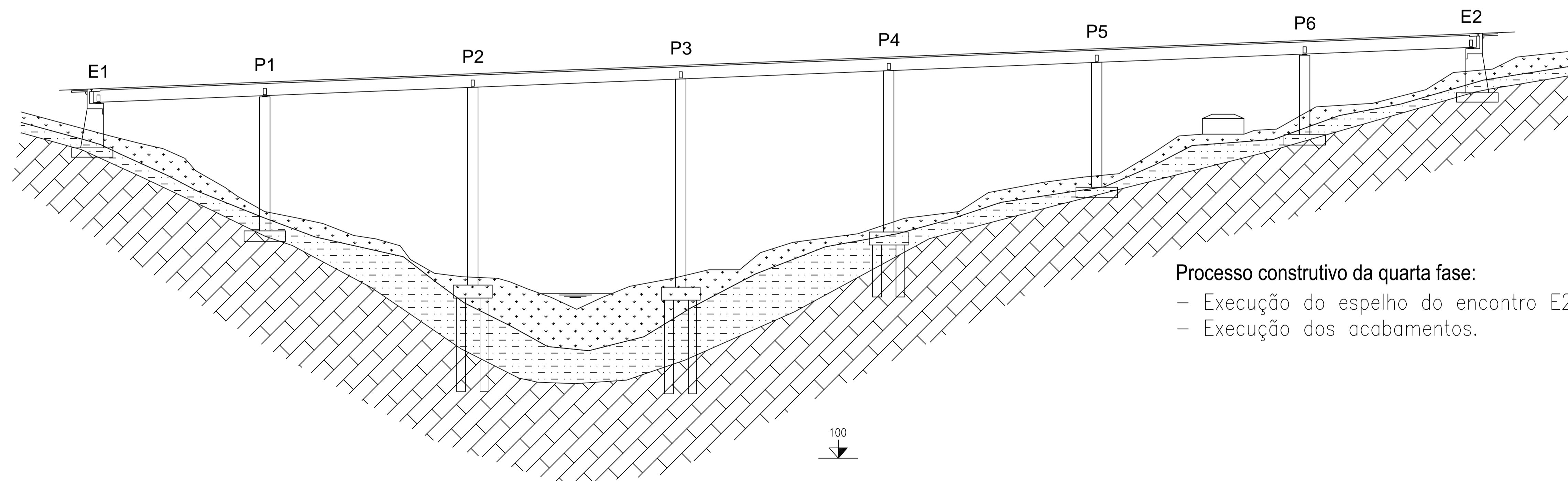
Quarta Fase ESCALA - 1:500
