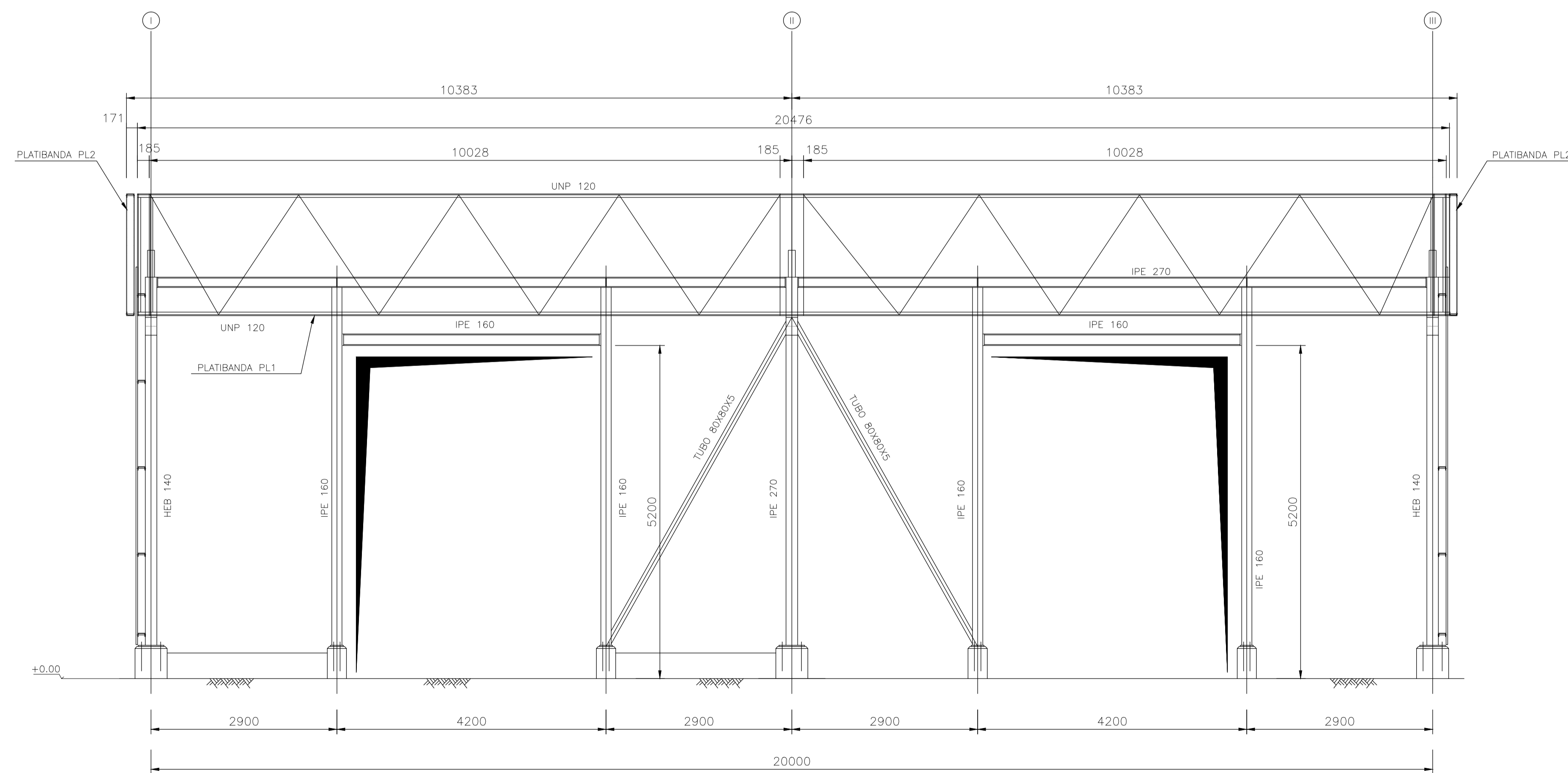
PÓRTICO-ALINHAMENTO A
