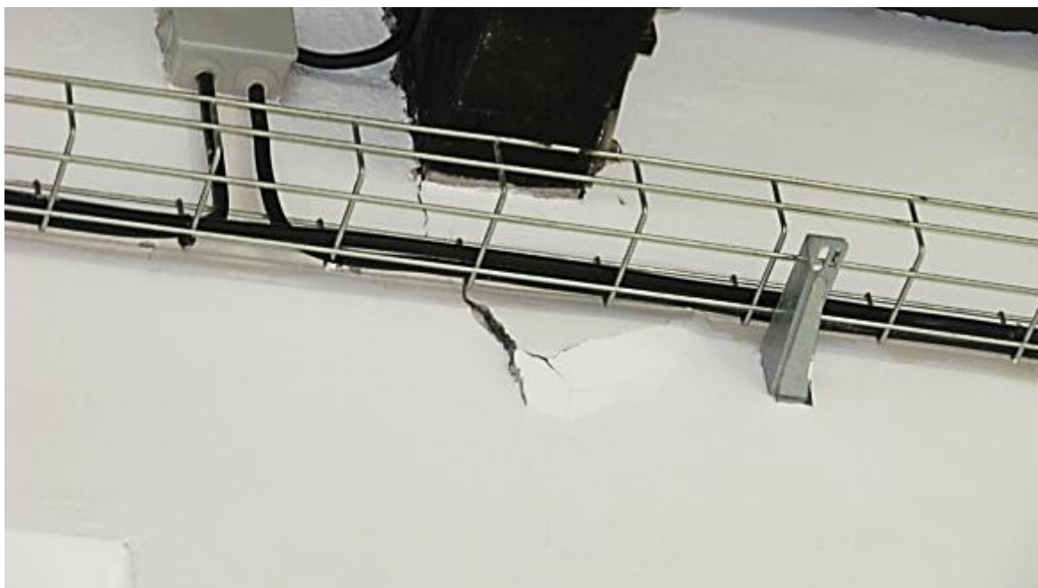
Figura V.1.2 – Centro de Atendimento Permanente em Seia (patologias do edifício) - Fendilhação em parede interior
