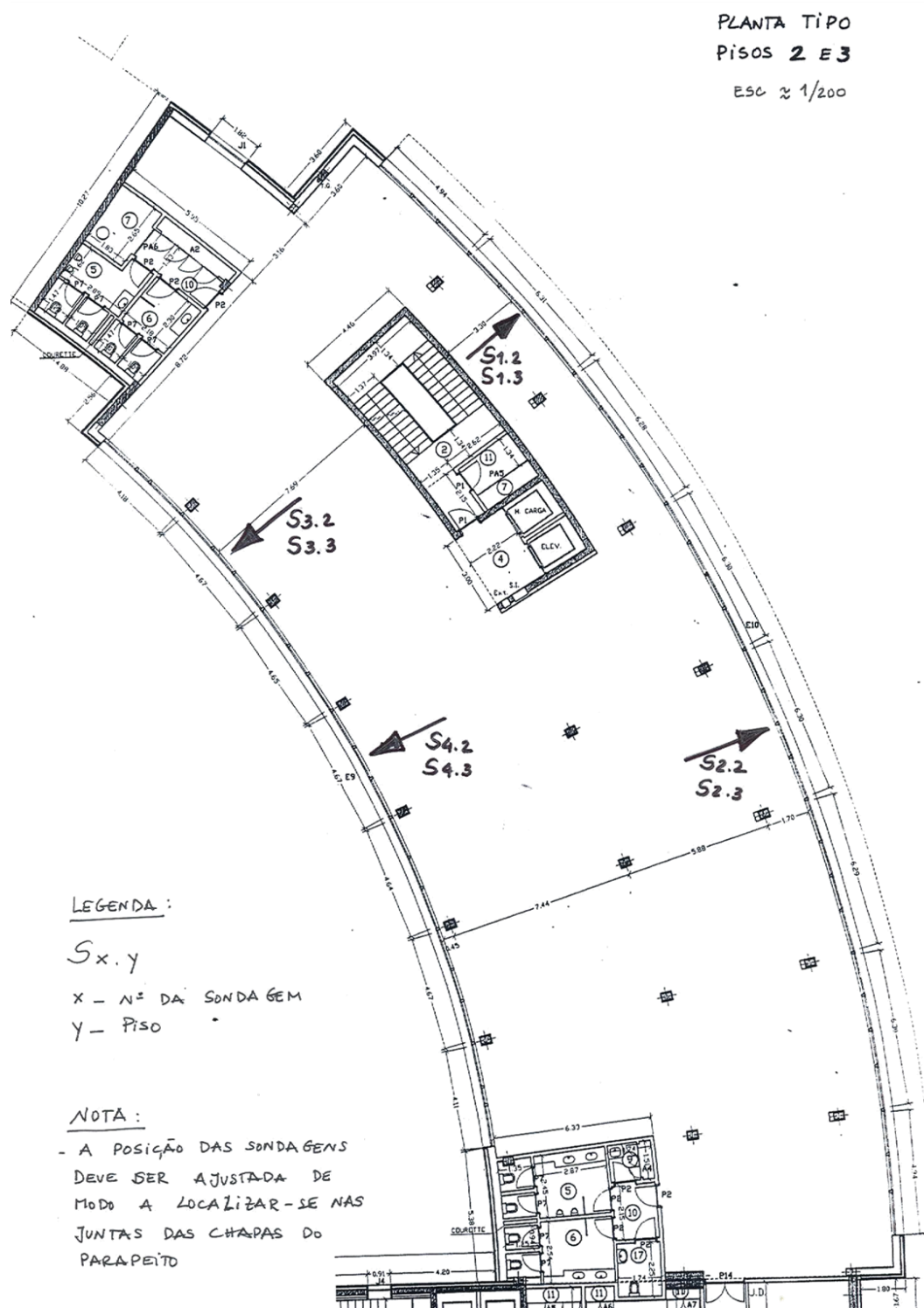
Figura II.1 – Edifício Sede de Escritórios em Coimbra - Localização em planta das sondagens
