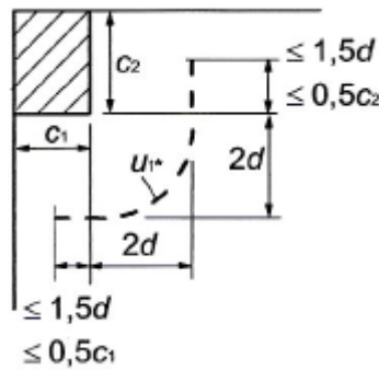
Fig. 20 - Primeiro perímetro de controlo reduzido ( u_1^* ) de um pilar de canto Fonte: (NP EN 1992-1-1, 2010)
