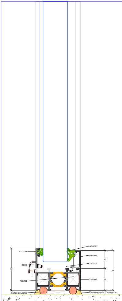
Pormenor 02 Escala 1:1
