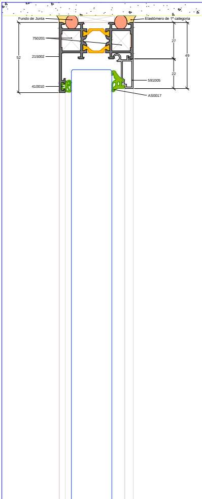
Pormenor 01 Escala 1:1
