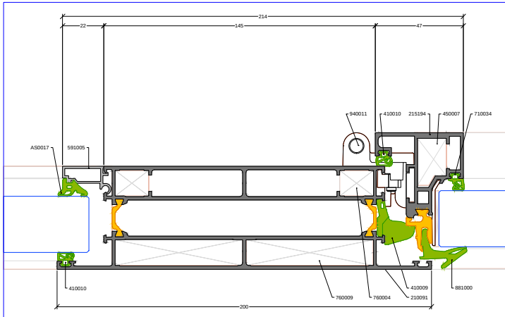
Pormenor 05 (opção prumo 210091) Escala 1:1
