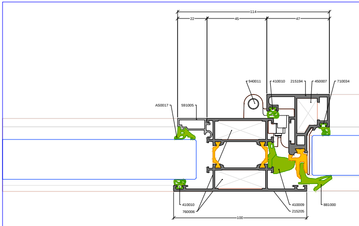
Pormenor 05 (opção prumo 215205) Escala 1:1
