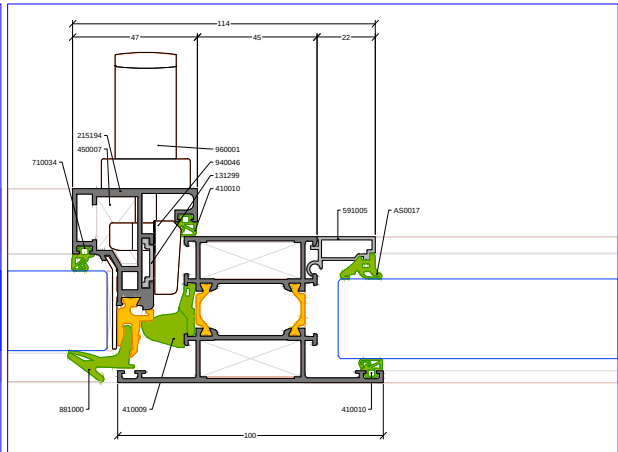
Pormenor 06 (opção prumo 215205) Escala 1:1
