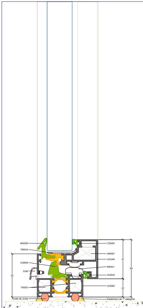
Pormenor 04 Escala 1:1
