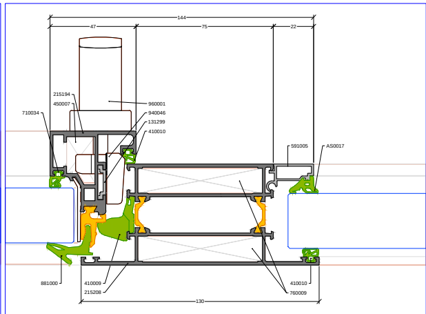
Pormenor 06 (opção prumo 215208) Escala 1:1
