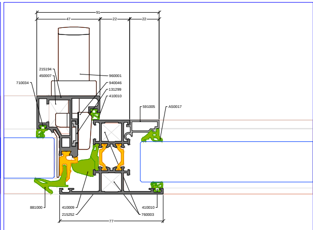
Pormenor 06 (opção prumo 215202) Escala 1:1
