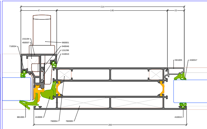
Pormenor 06 (opção prumo 210091) Escala 1:1
