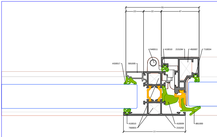
Pormenor 05 (opção prumo 215202) Escala 1:1
