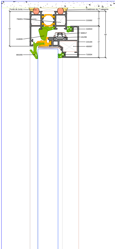
Pormenor 03 Escala 1:1
