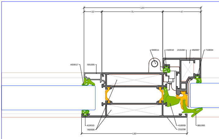
Pormenor 05 (opção prumo 215208) Escala 1:1
