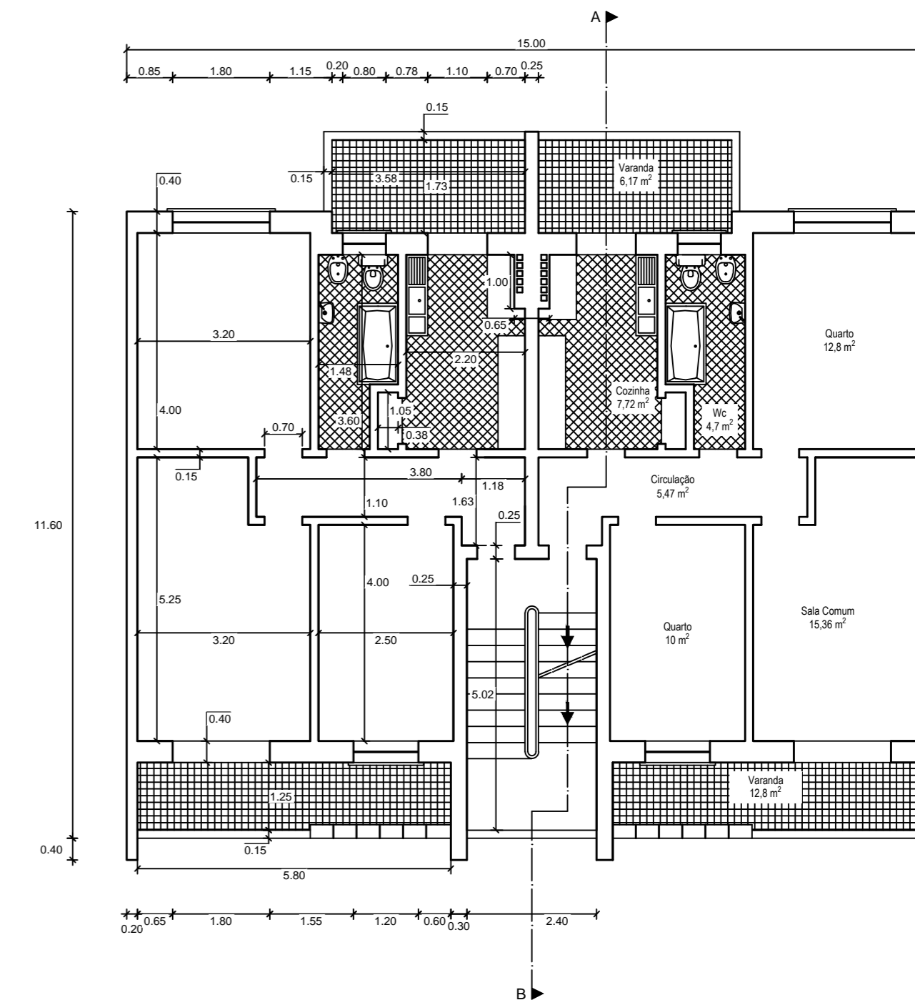
Planta dos Andares
