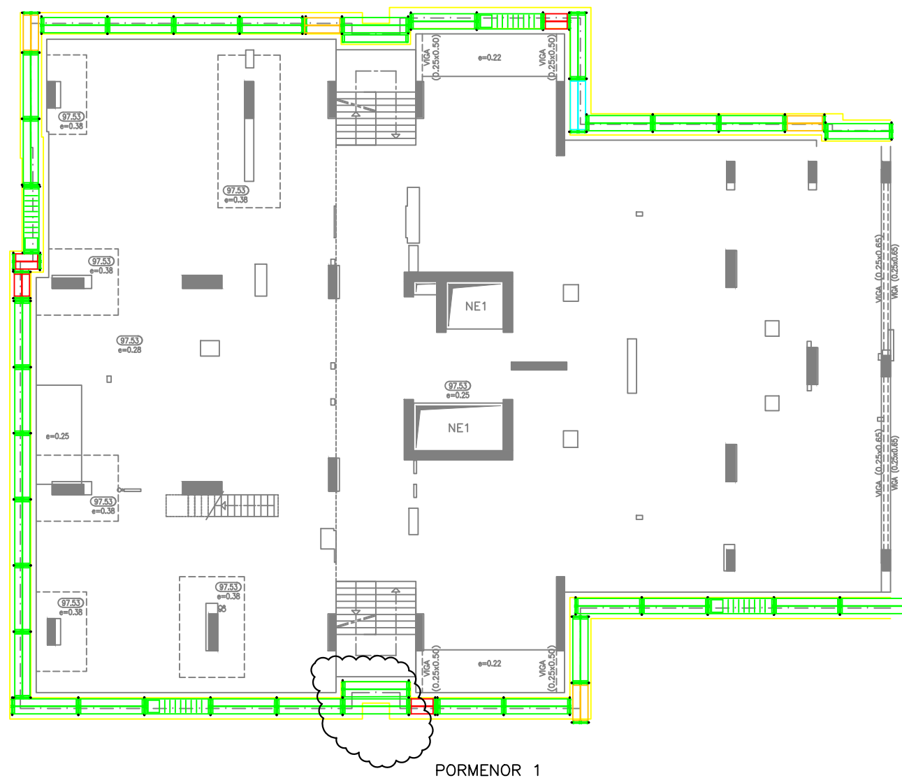
TORRE A PLANTA DO PISO 0 ao PISO 5 Esc. 1:100
