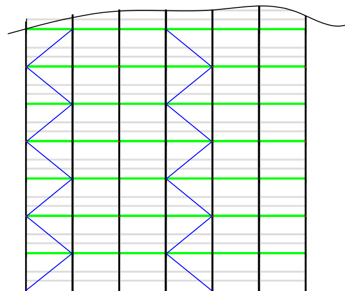
TORRE A ALÇADO DO PISO 0 ao PISO 5 Esc. 1:100
