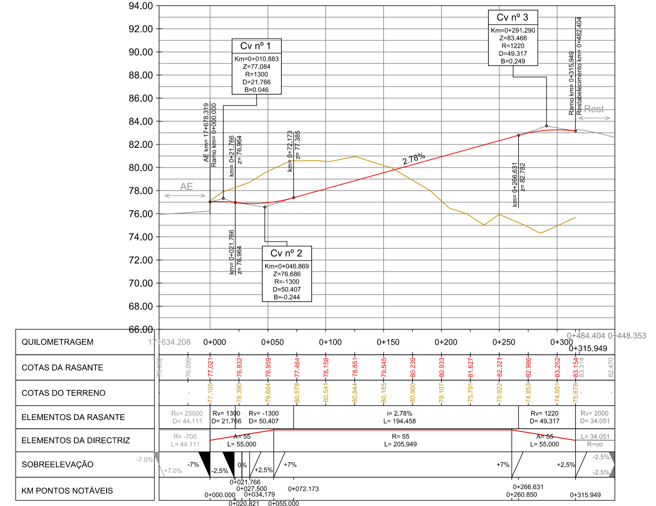
Perfil Longitudinal do Ramo
