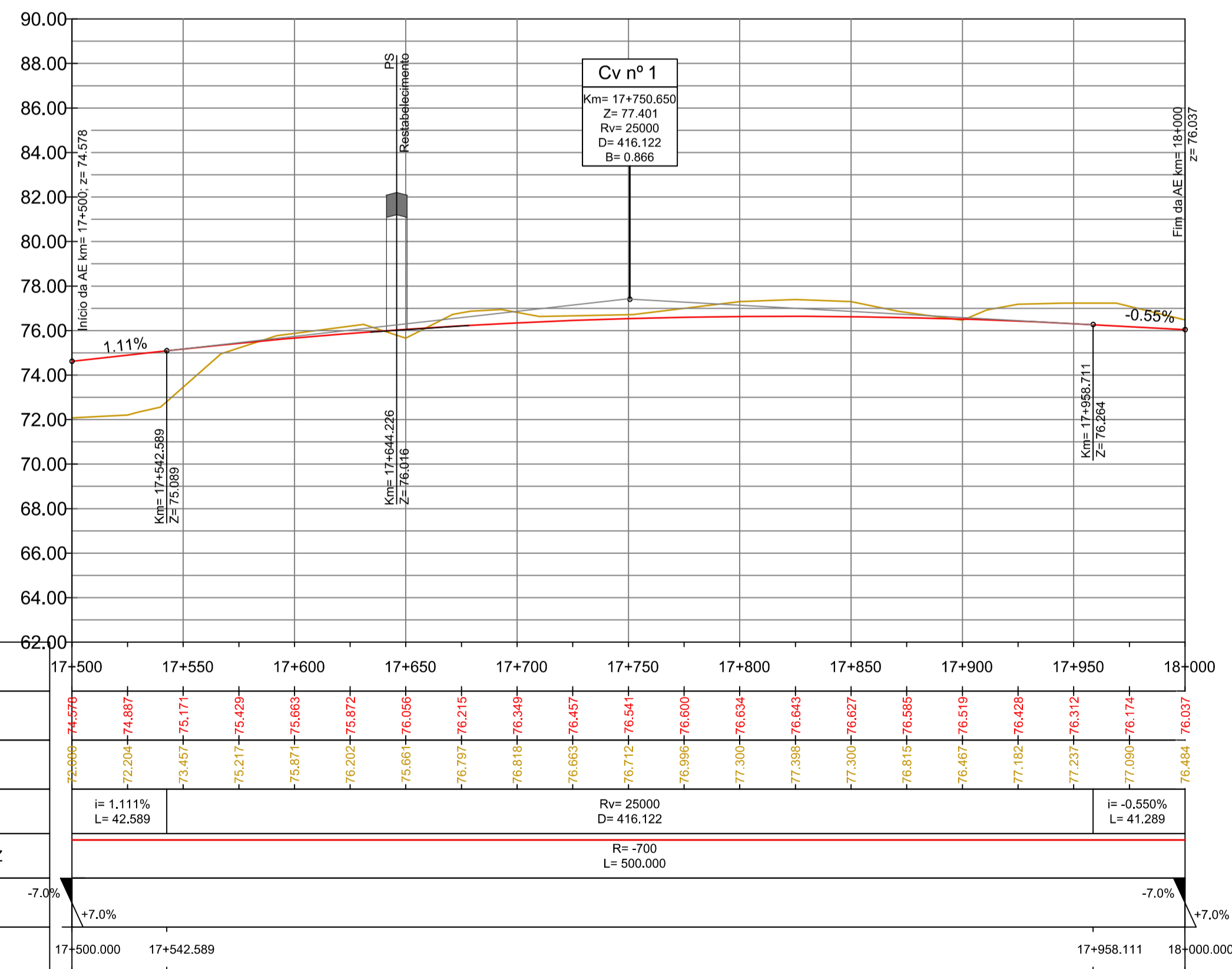
Perfil Longitudinal da Autoestrada
