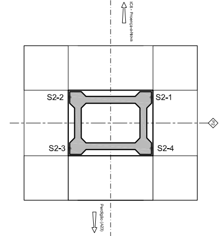
SAPATA DO PILAR P2 - INSTRUMENTAÇÃO
