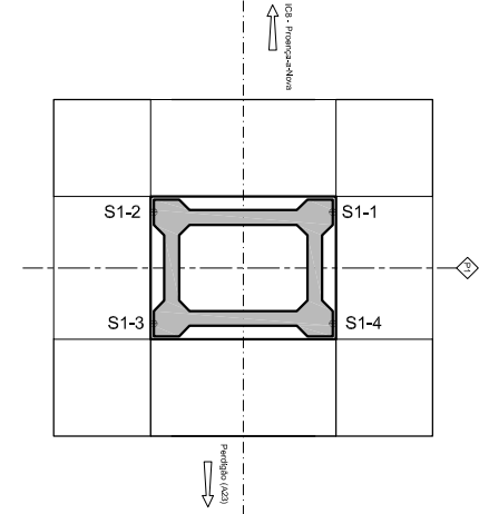
SAPATA DO PILAR P1 - INSTRUMENTAÇÃO
