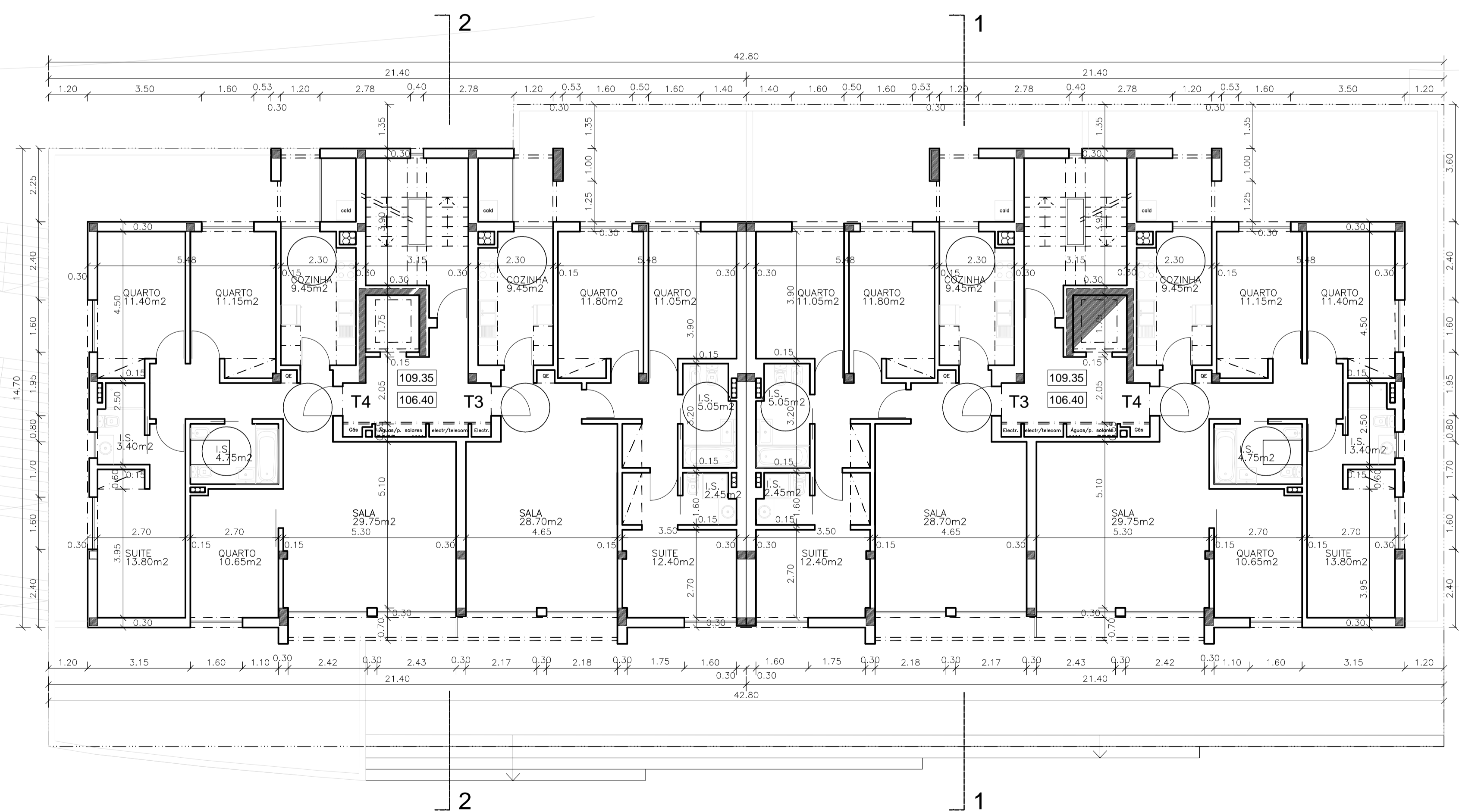
PLANTA DO PISO TIPO
