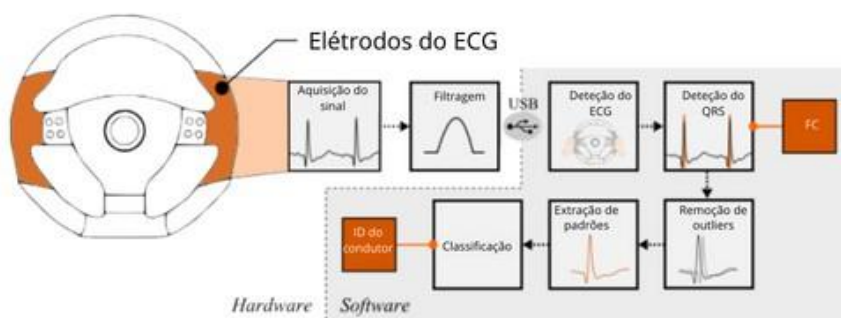
Figura 14 Arquitetura do sistema CardioWheel. Adaptado (32)
