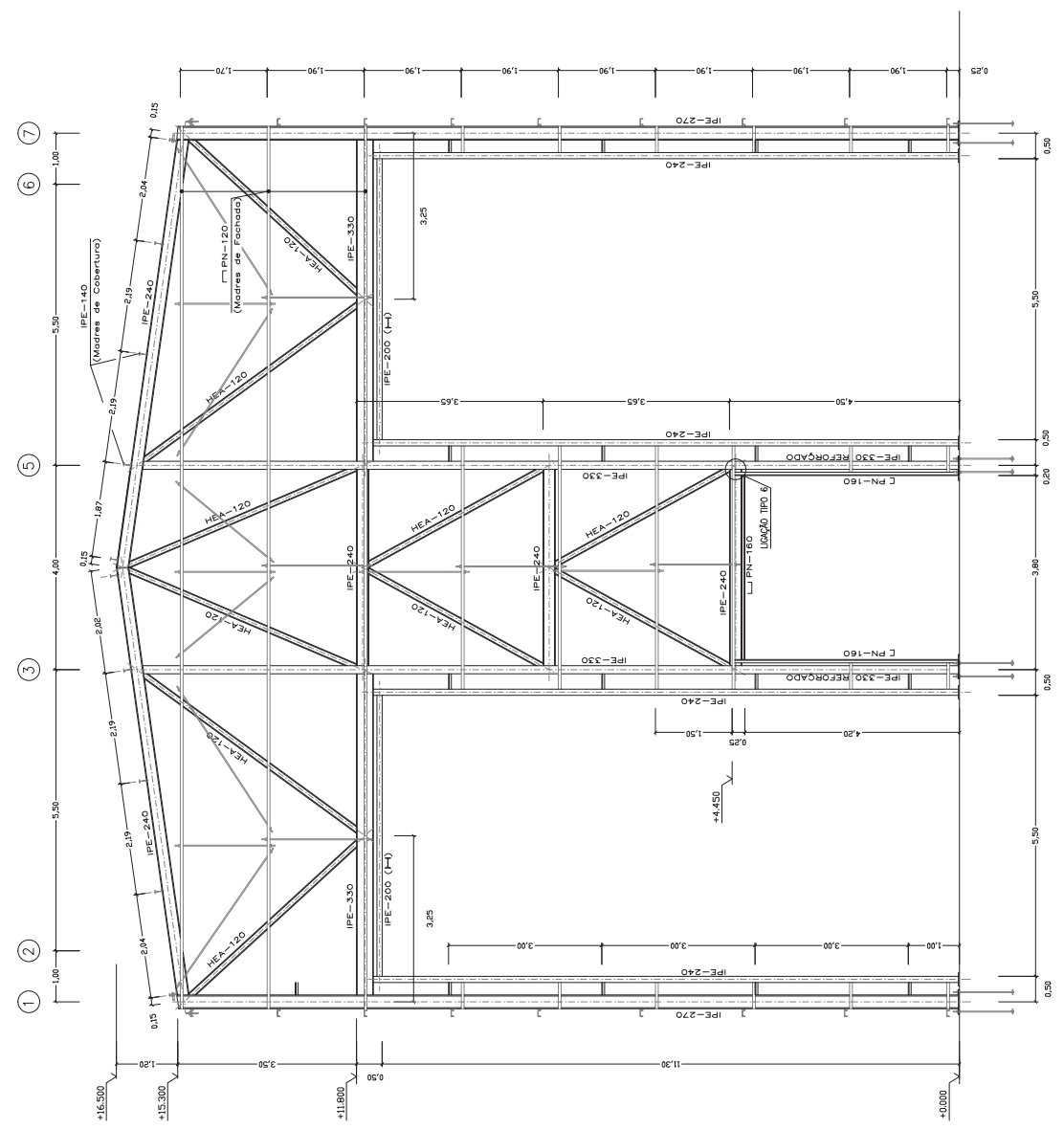
PÓRTICO H ESC: 1:50
