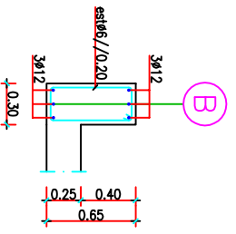
SECÇÃO 16-16
