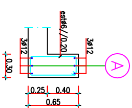
SECÇÃO 14-14
