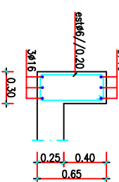
SECÇÃO 12-12
