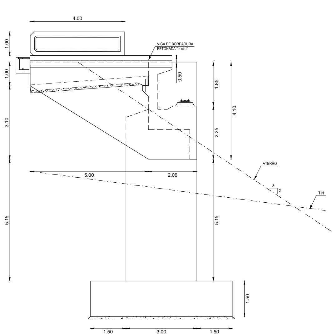
ALÇADO LATERAL ESQUERDO (A1-1:50, A3-1:100)
