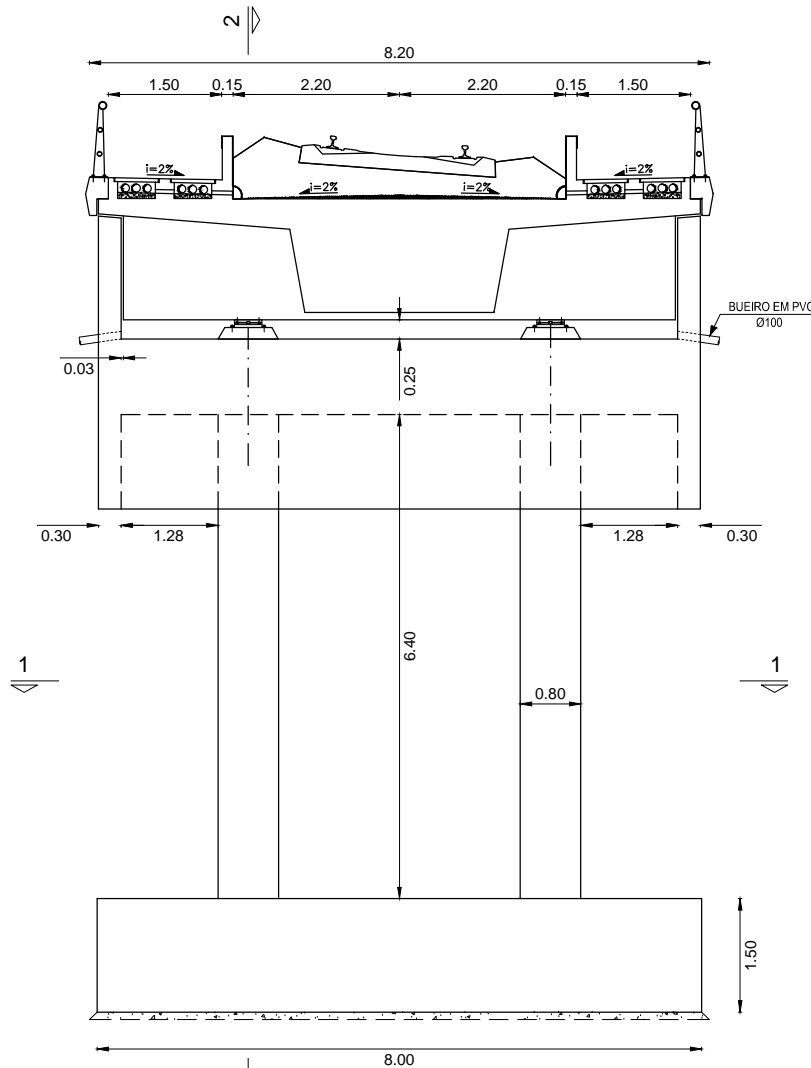
ALÇADO FRONTAL (A1-1:50, A3-1:100)
