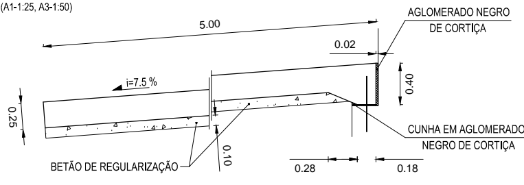
LAJE DE TRANSIÇÃO (A1-1:25, A3-1:50)
