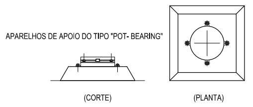
APARELHOS DE APOIO (A1-1:20, A3-1:40)
