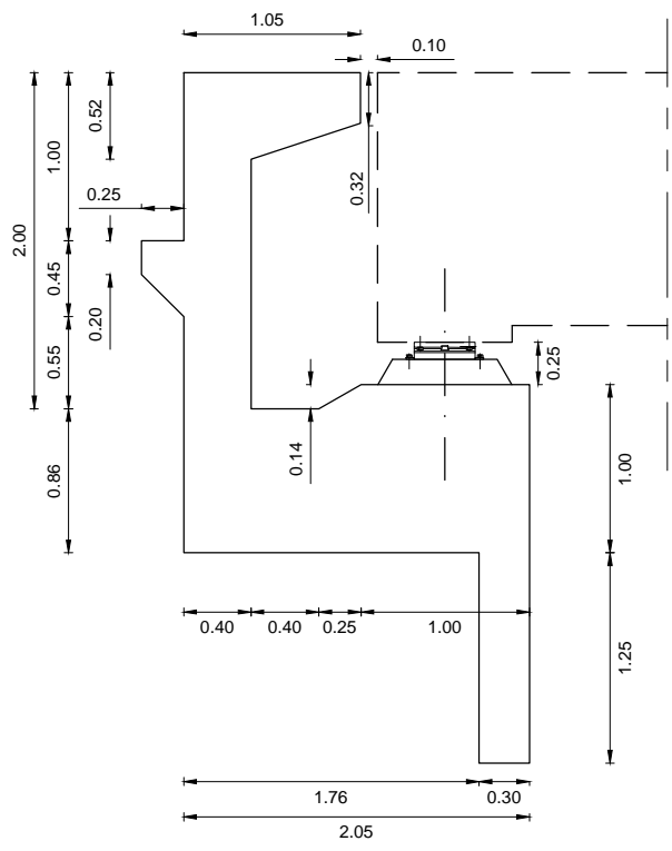
VIGA DE ESTRIBO (A1-1:25, A3-1:50)
