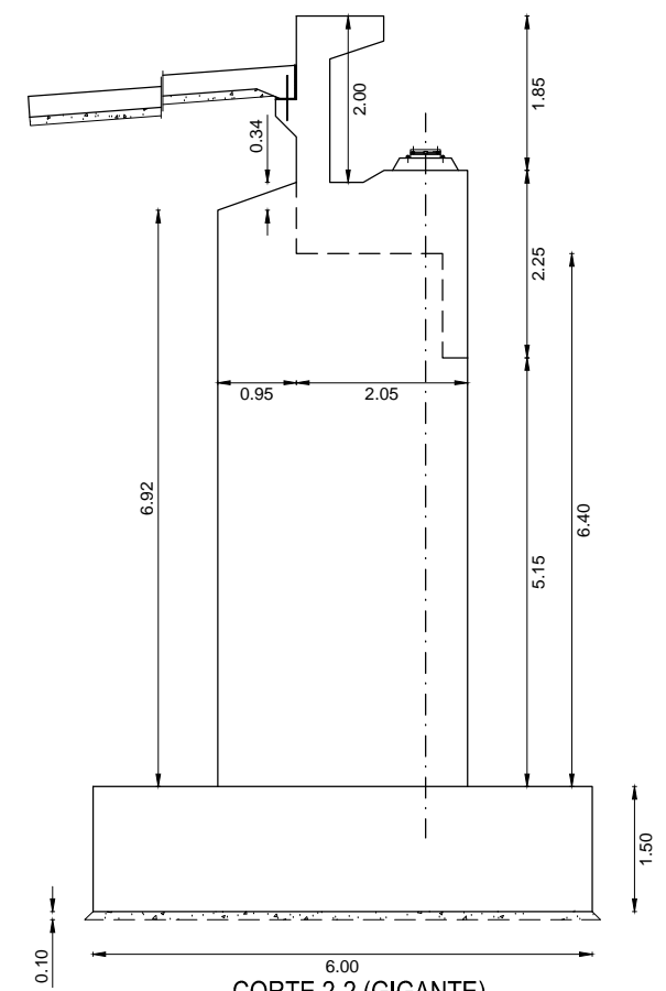
CORTE 2-2 (GIGANTE) (A1-1:50, A3-1:100)
