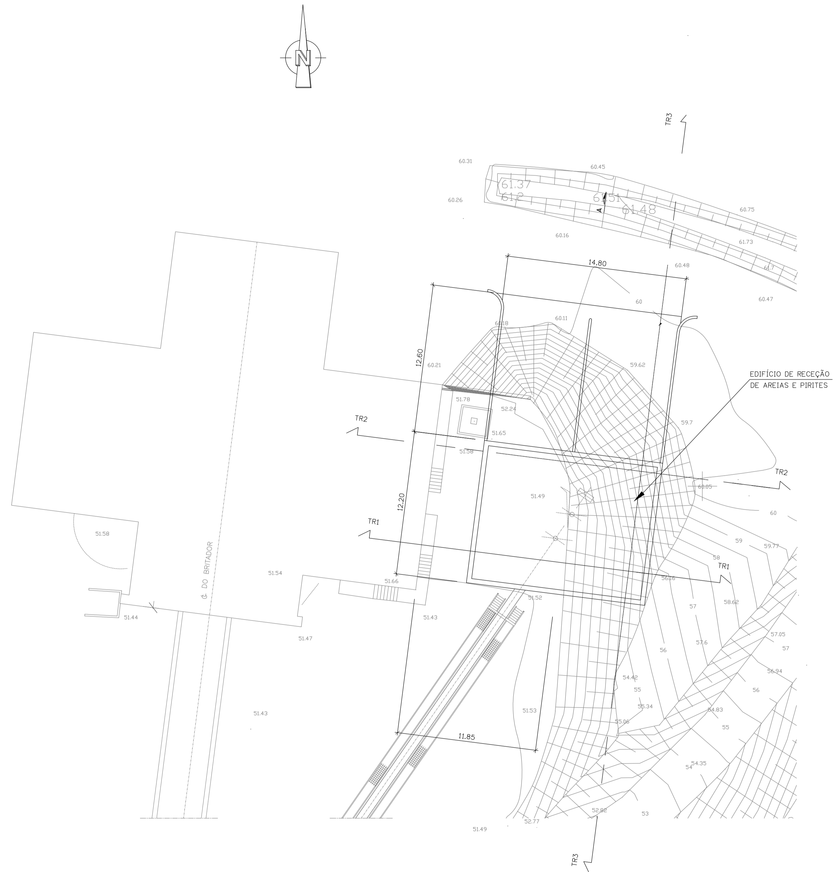
PLANTA DE IMPLANTAÇÃO DO EDIFÍCIO
